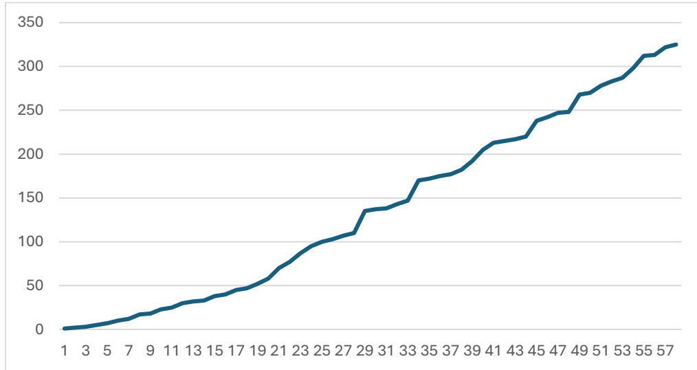
Diagramme 8 : Facteurs multiplicatifs du nombre 24 associés à la différence entre les carrés des nombres d'une paire de nombres premiers jumeaux (en usant des données de la séquence A002822)
