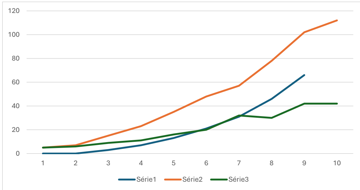
Diagramme 3 : Comparaison entre le nombre de faux positifs, de semi-premiers et de nombres premiers situés entre les carrés d'une paire de nombres premiers jumeaux
