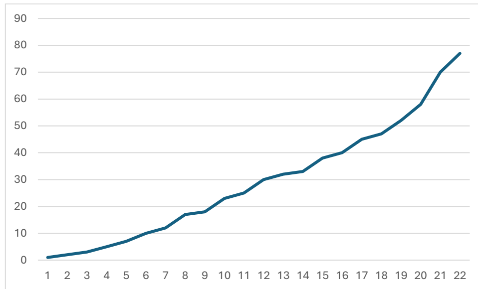
Diagramme 7 : Facteurs multiplicatifs du nombre 24 associés à la différence entre les carrés des nombres d'une paire de nombres premiers jumeaux
