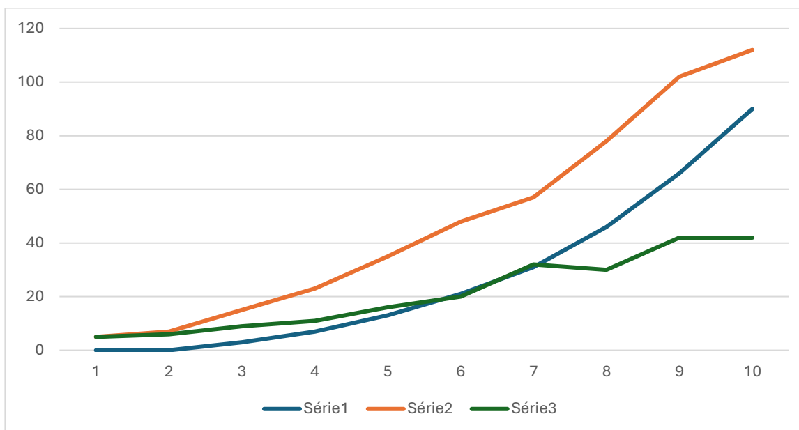
Diagramme 4 : Courbe des faux positifs avec un nombre de 90 items (Série 1)
