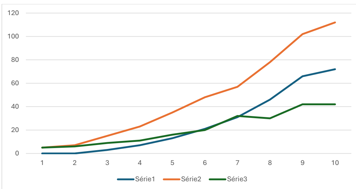
Diagramme 5 : Courbe des faux positifs avec un nombre de 72 items (Série 1)
