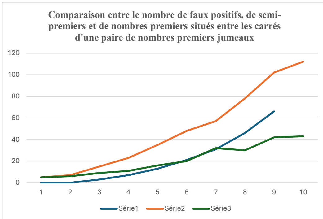
Diagramme 3 : Comparaison entre le nombre de faux positifs, de semi-premiers et de nombres premiers situés entre les carrés d'une paire de nombres premiers jumeaux
