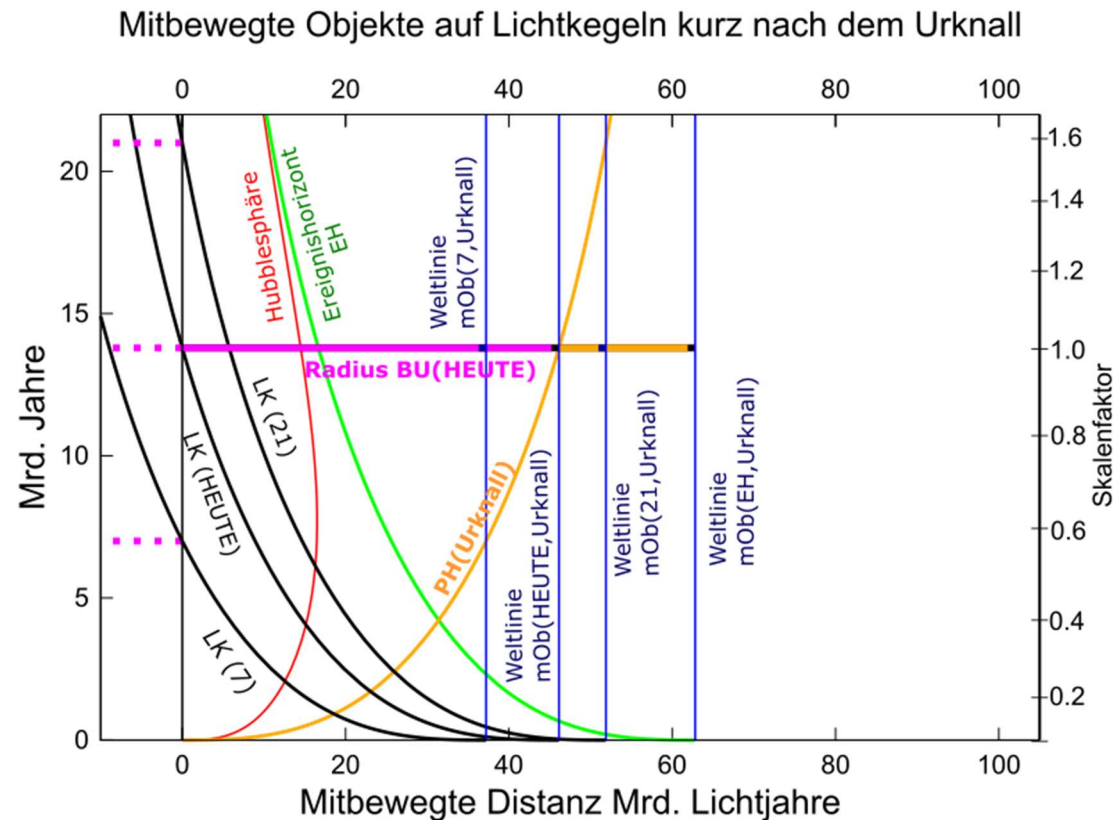
Abbildung 4: Mitbewegte Objekte auf Lichtkegeln und dem EH kurz nach dem Urknall - zeitäquidistant (t) – mitbewegte Abstände (d mitbewegt)
