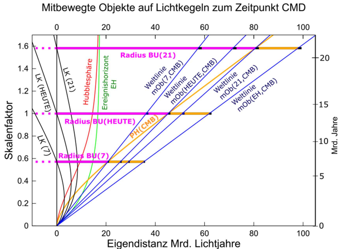
Abbildung 2: Mitbewegte Objekte auf Lichtkegeln und dem EH zum Zeitpunkt CMB – Skalenfaktor-äquidistant (a) – physikalische Abstände (d)
