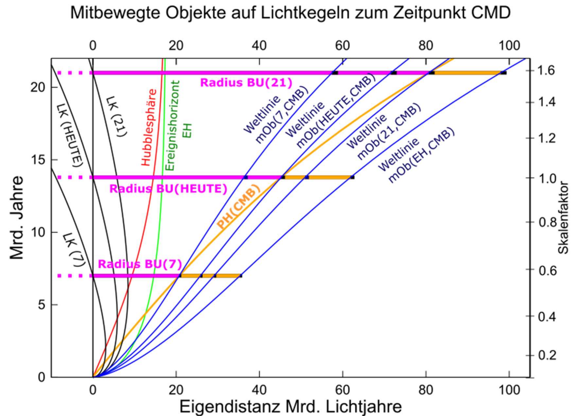
Abbildung 1: Mitbewegte Objekte auf Lichtkegeln und dem EH zum Zeitpunkt CMB - zeitäquidistant (t) – physikalische Abstände (d)
