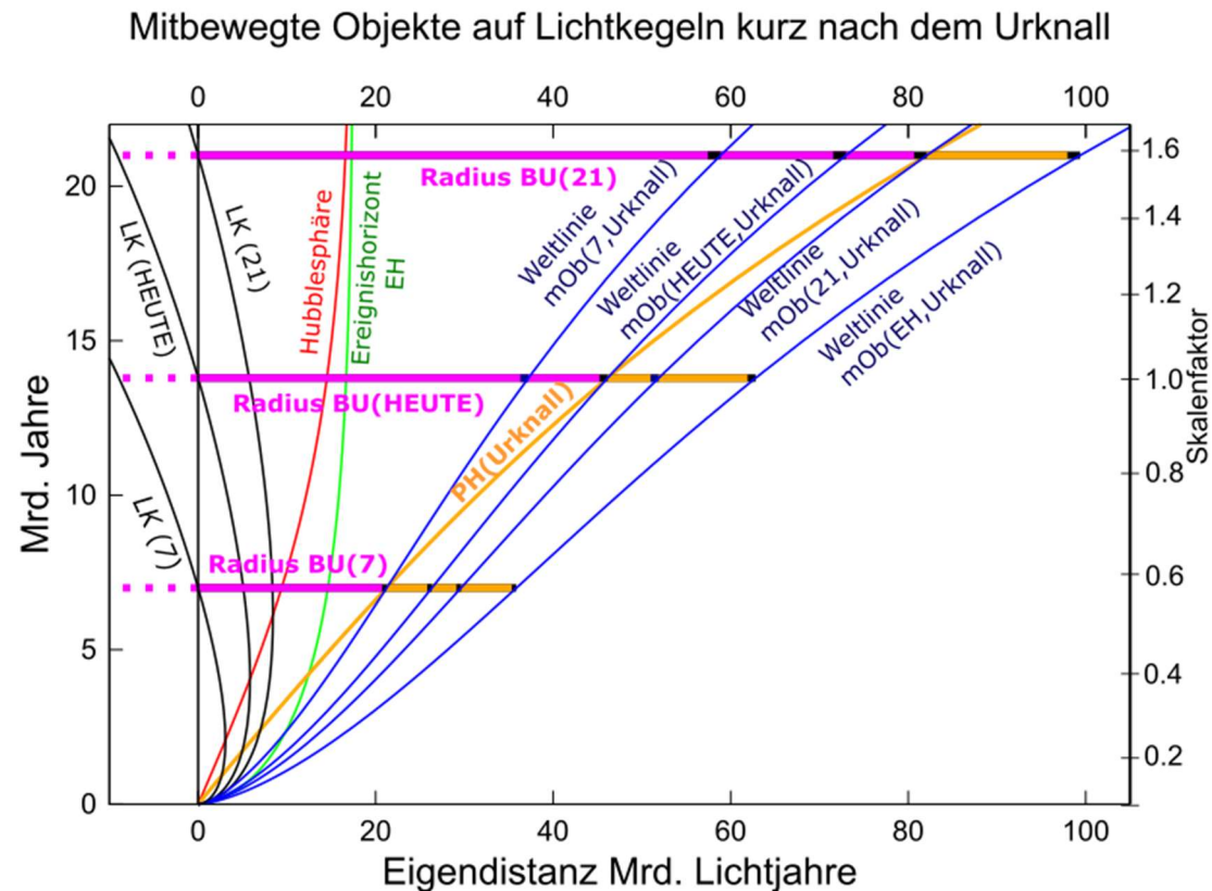
Abbildung 3: Mitbewegte Objekte auf Lichtkegeln und dem EH kurz nach dem Urknall - zeitäquidistant (t) – physikalische Abstände (d)
