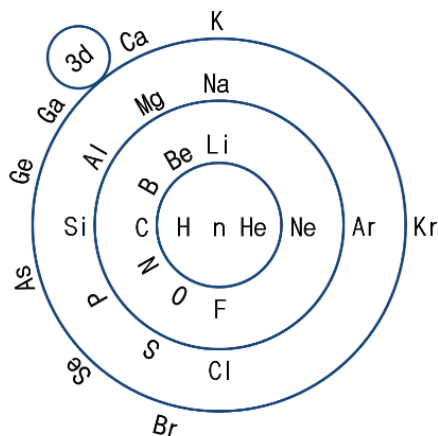
图 2. 小型版环形元素周期表
