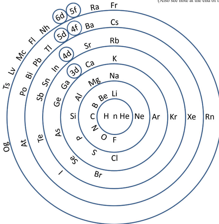
图 1. 环形元素周期表
