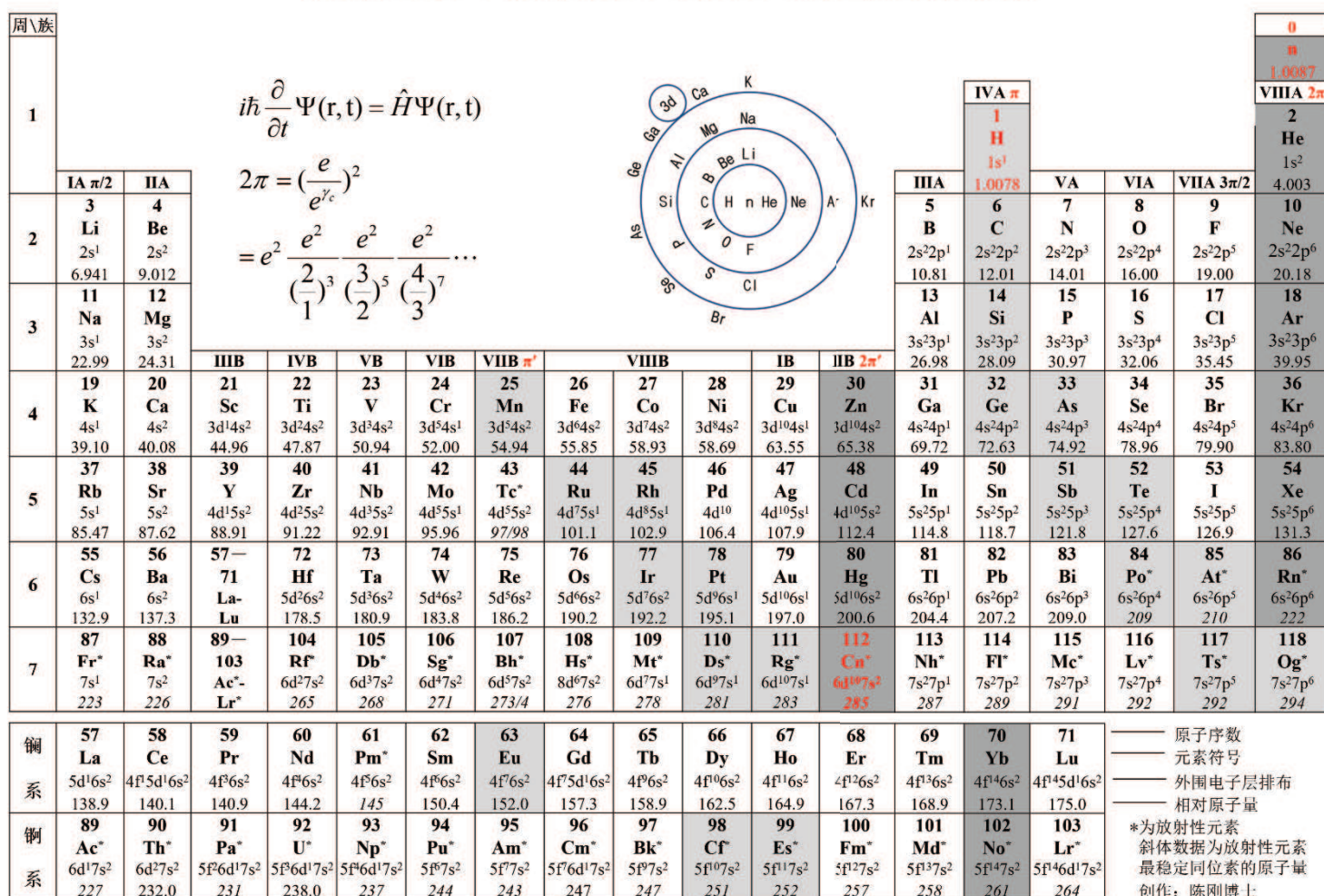
图3. 改进版元素周期表
