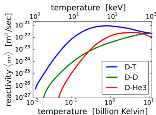
图 8. 核聚变条件
