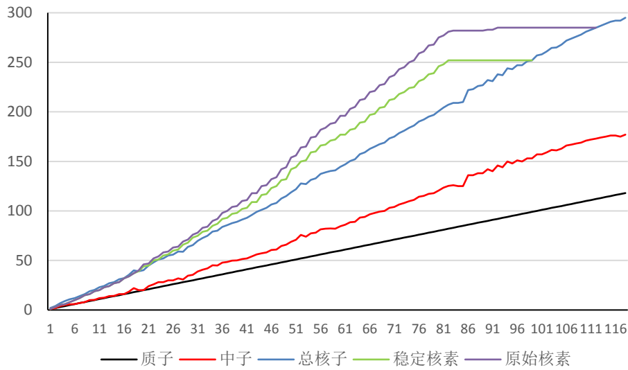
图 10. 元素的质子、中子、总核子、原始核素和稳定核素的数量对比图
