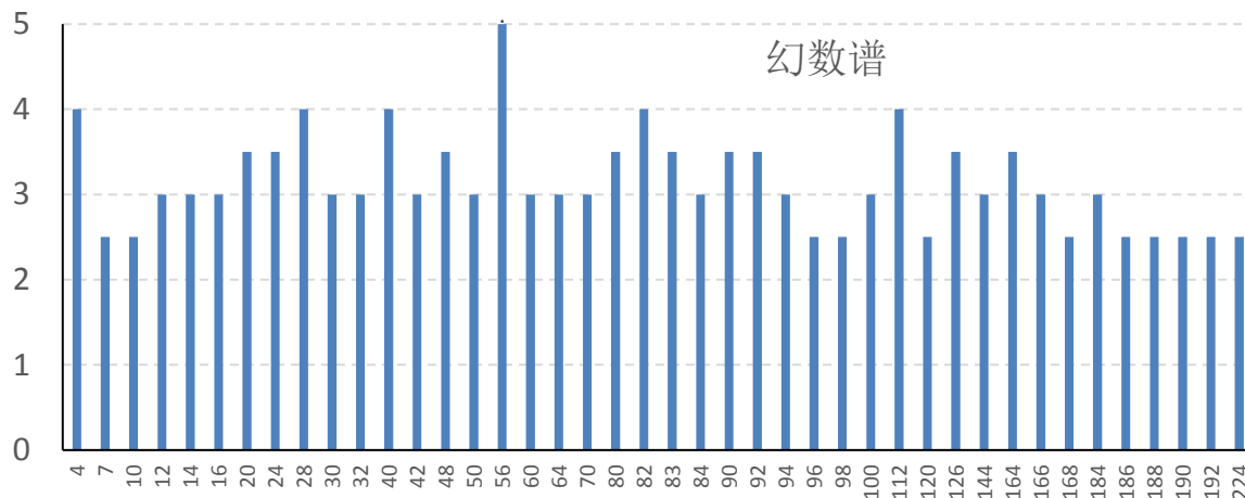
图 2. 幻数谱
