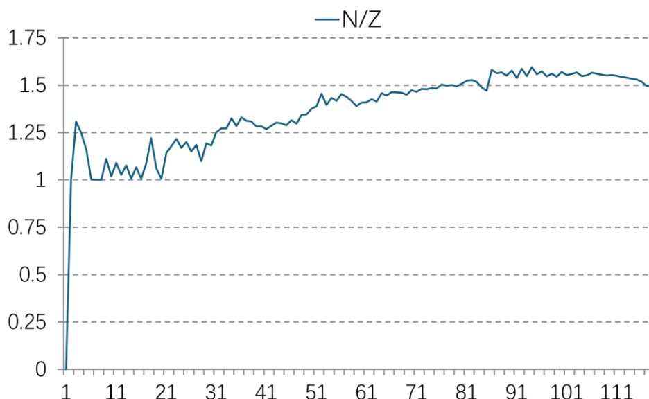
图 6. 元素的质子数和中子数比例图
