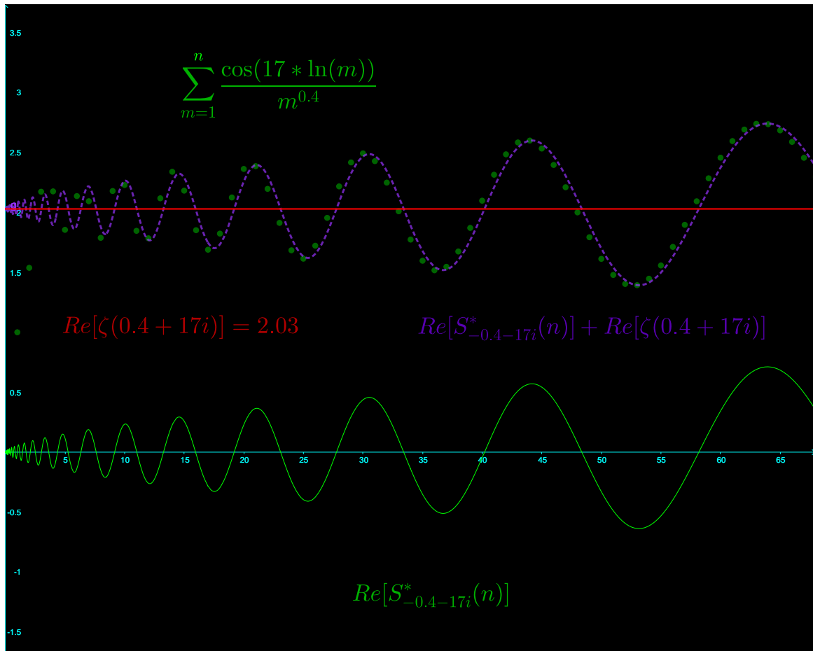
Figura 3: Representación gráfica de las funciones Re[S_{-s}^*(n)] y la serie \sum_{m=1}^n \frac{1}{m^{Re[s]}} \cos(Im[s] * \ln m) que oscila respecto a su valor medio Re[\zeta(s)] , con amplitud creciente cuando Re[s] \leq 1 y amplitud decreciente cuando Re[s] > 1
