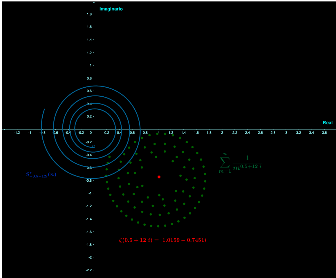
Figura 2: Gráfica en el plano complejo de las espirales dadas por la función S_{-s}^*(n) (en color azul), y la serie \sum_{m=1}^n \frac{1}{m^s} (en color verde) y el centro de la espiral \zeta(s) (en color rojo).
