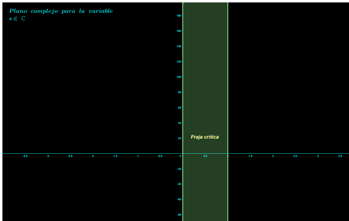
Figura 5: Franja crítica en el Plano complejo, para la variable s \in \mathbb{C} , donde no es posible determinar \zeta(s) , con la Ecuación Funcional de Riemann.
