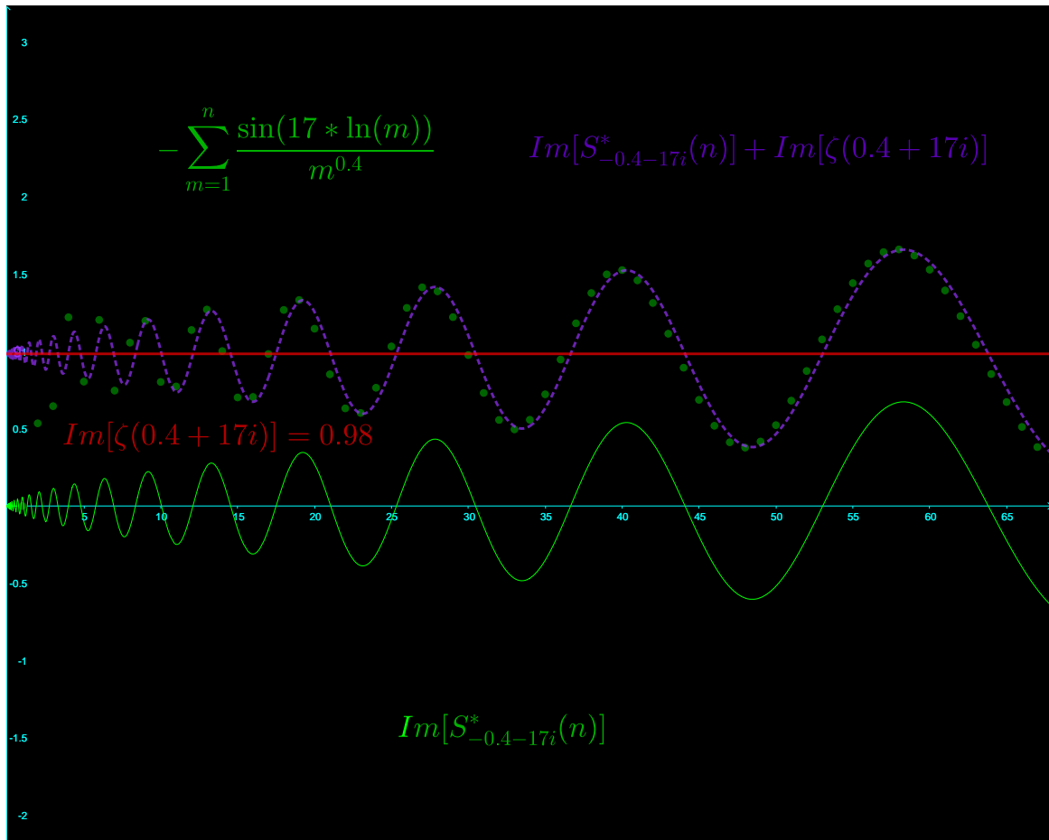
Figura 4: Representación gráfica de las funciones Im[S_{-s}^*(n)] y la serie \sum_{m=1}^n \frac{1}{m^a} \sin(-Im[s] * \ln m) que oscila respecto a su valor medio Im[\zeta(s)] , con amplitud creciente cuando Re[s] \leq 1 y amplitud decreciente cuando Re[s] > 1
