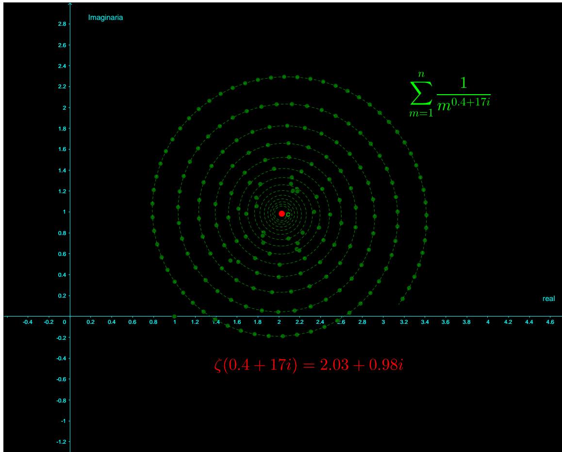
Figura 1: Ejemplo de espiral logarítmica de la serie \sum_{m=1}^n \frac{1}{m^s} para s = 0,4 + 17i donde \zeta(s) es el centro de la espiral.
