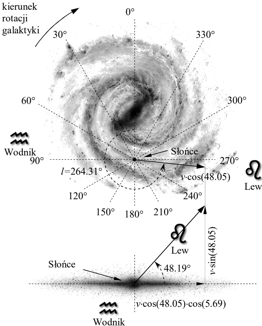
Rys. 3. Prędkość Układu Słonecznego względem eteru.
