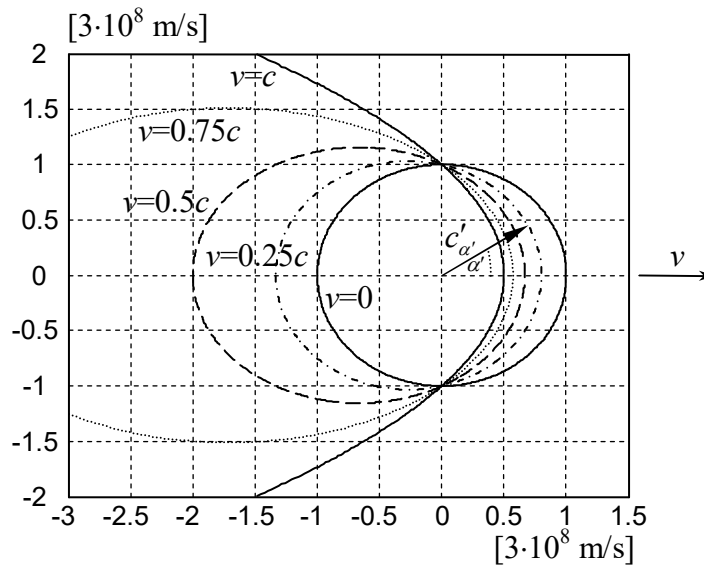
Rys. 4. Jednokierunkowa prędkość światła c'_{s\alpha'} przewidywana przez STE w układzie inercyjnym dla v = 0, 0.25c, 0.5c, 0.75c, c [źródło [22]].
