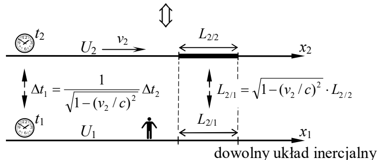
Rys. 1. Podobieństwa pomiędzy STW oraz STE ( \psi(v) = 1 ) [źródło [21]].
