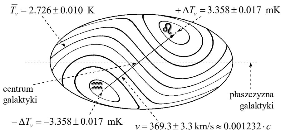
Rys. 2. Dipolowa anizotropia mikrofalowego promieniowania tła pokazana w projekcji Hammer'a-Aitoff [źródło [23]].
