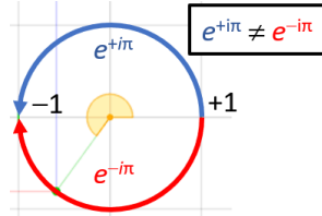
Figure 10: e^{+i\pi} \neq e^{-i\pi}
