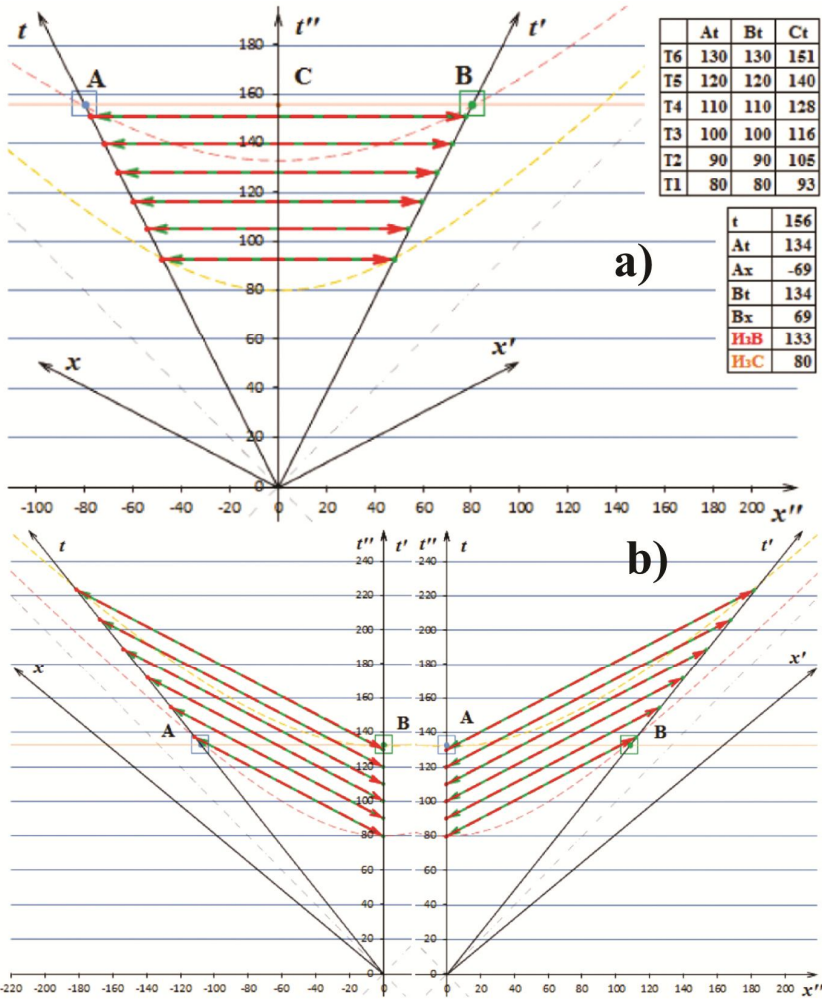
Рис.3.3. Многократный обмен сверхсветовыми сигналами с точки зрения средней системы и систем покоя A и B [20].
