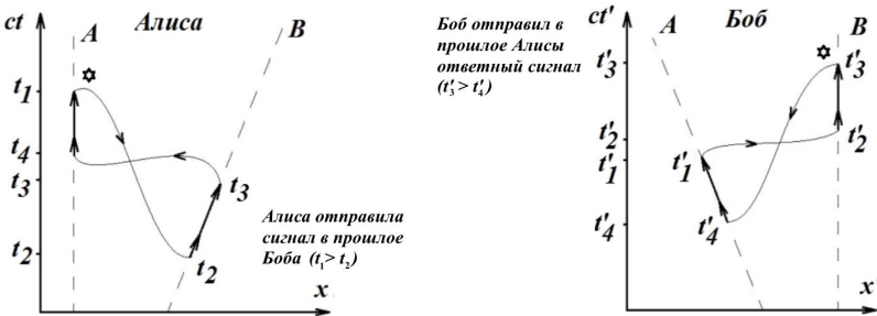
Рис.4.5. Обмен сверхсветовыми сигналами на диаграммах Минковского
