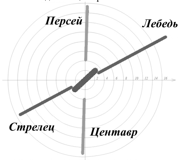
Рис.6.13. Вид рукавов галактики Млечный Путь в момент их возникновения. Кадр из анимации [20]
