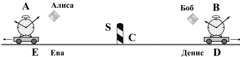
Рис.4.15. Алиса и Боб бросили нелокальные кубики
