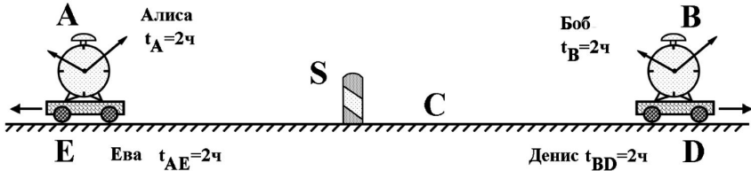
Рис.4.3. Алиса поравнялась с Евой, а Боб с Денисом. Что видят на часах Алисы и Боба все участники?
