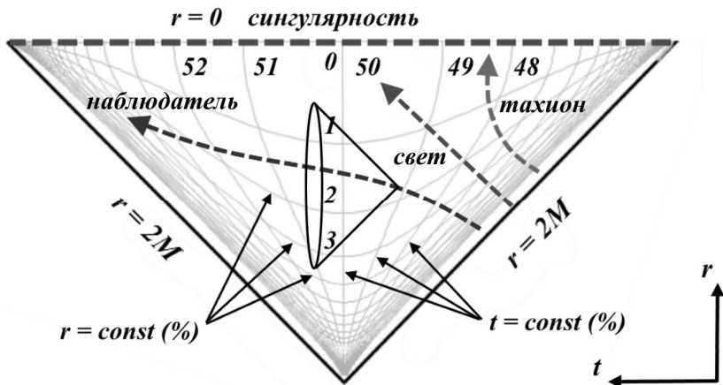
Рис.6.18. Сингулярный треугольник Черной дыры – верхняя часть диаграммы коллапса нейтронной звезды
