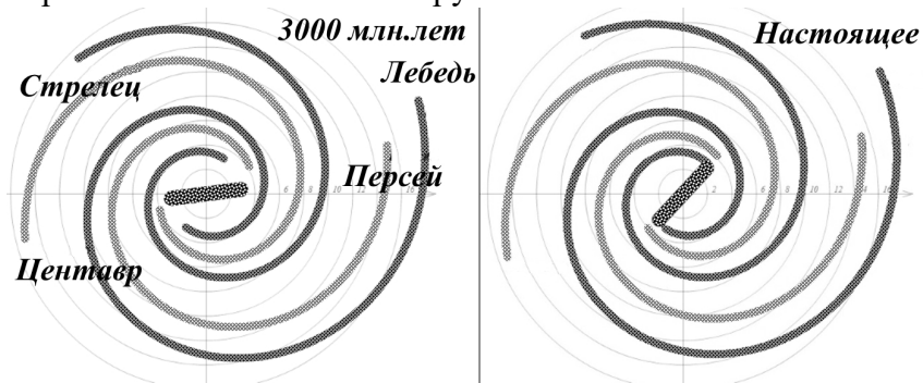
Рис.6.14. Изображение галактики Млечный Путь с рукавами, образованными за 3 млрд. лет из двух пар джетов (слева) и нынешнее её представление (справа). Кривая вращения – спрямляющая Рукав Лебеда.
