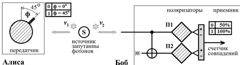
Рис.2.3. Схема квантового нелокального семафора
