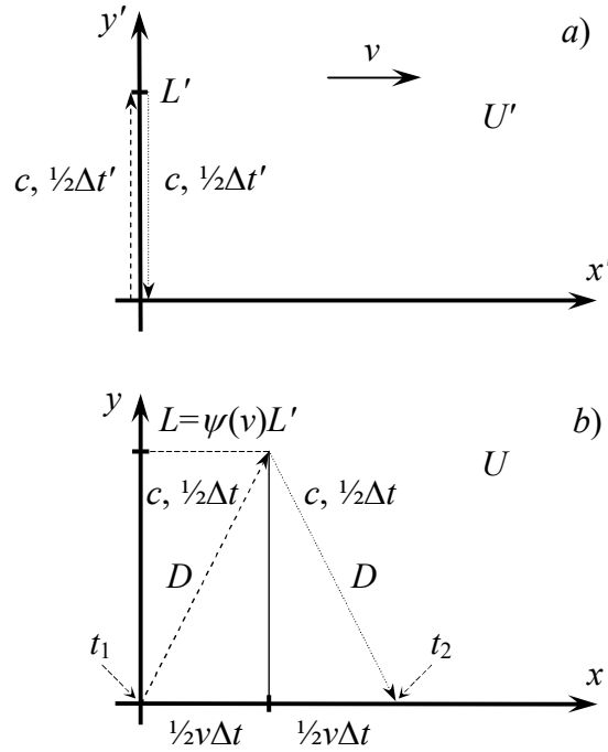
Рис. 2. Путь, проходимый светом, видимый из двух систем отсчета. a) инерциальная система отсчета U' , b) универсальная система отсчета U .
