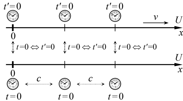
Рис. 8. Синхронизация часов внешним методом ( e(v) = 0 ).
