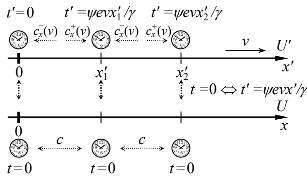
Рис. 9. Синхронизация часов внешним методом ( e(v) \neq 0 ).
