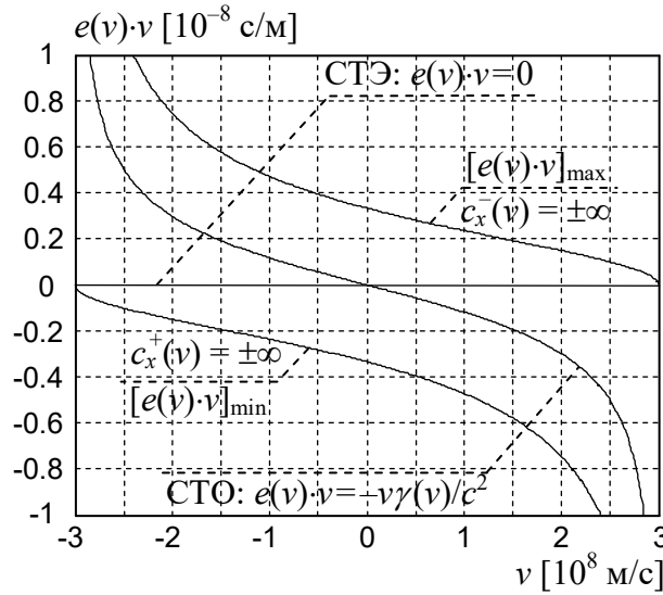
Рис. 4. Область значений функции e(v) \cdot v , для которой не наблюдается мнимого возвращения света во времени.
