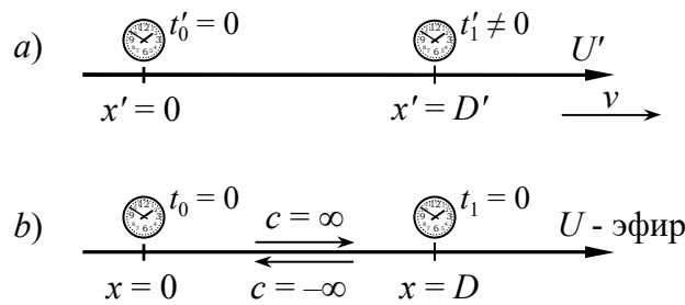
Рис. 7. Измерение скорости света в инерциальной системе отсчета при рассинхронизированных часах в ней, а также в универсальной системе отсчета (эфире) при бесконечной скорости света.
