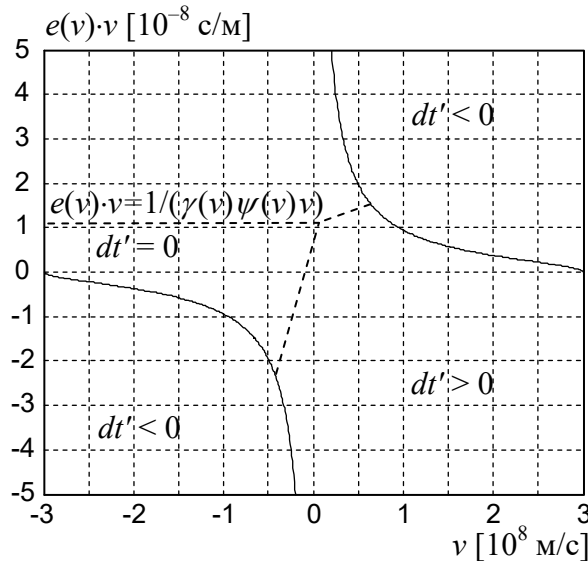
Рис. 11. Влияние значения параметра e(v) на измерение времени в движущейся инерциальной системе наблюдателем из универсальной системы отсчета ( dt > 0 и \psi(v) = 1 ).
