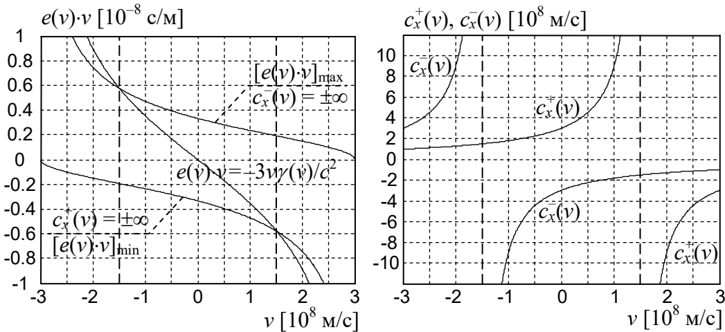
Рис. 5. Однонаправленная скорость света в вакууме как функция скорости v для e(v) \cdot v = -3v\gamma(v)/c^2 .
