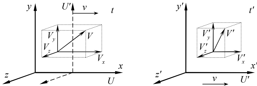
Рис. 3. Движение, видимое из универсальной и инерциальной систем отсчета.
