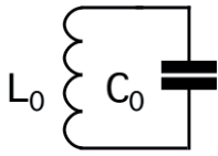
Bild 6 Ersatzschaltung eines statischen MLE
