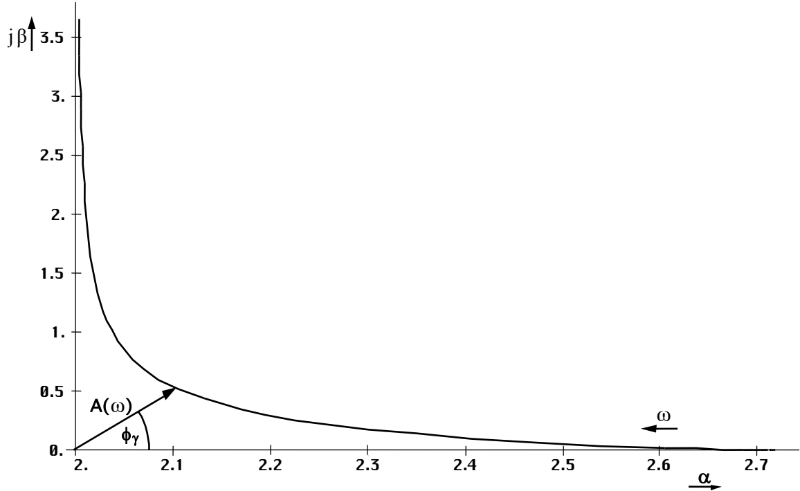
Bild 16 Frequenzgangsortskurve
