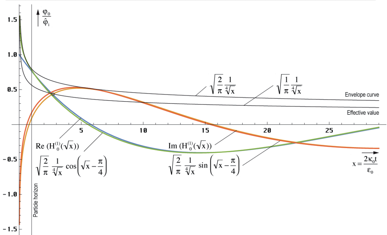
Bild 14 Verlauf von magnetischem Fluß sowie der Nähungs- und Hüllkurvenfunktionen in der Nähe der Singularität
