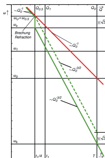
Bild 68a Einkopplungsprozeß
