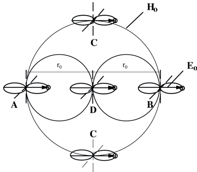
Bild 4 Anordnung der MLE an einer Feldlinie in x-Richtung bei kubisch flächenzentriertem Gitter
