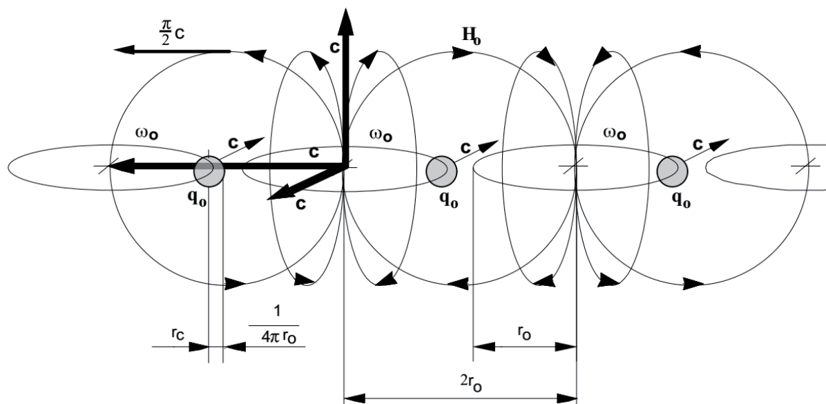
Bild 2 MINKOWSKISCHE Linienelemente Abmessungen und Kopplung untereinander
