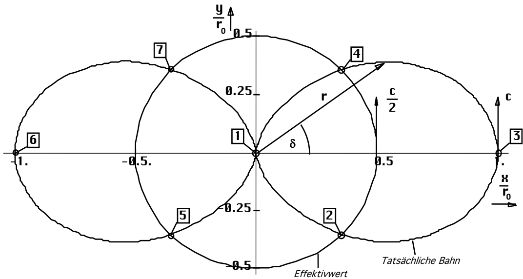
Bild 8 Bahnverlauf in der xy-Ebene
