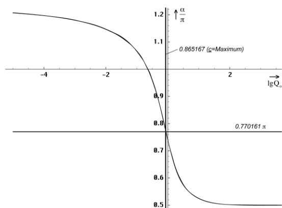
Bild 142 Winkel \alpha als Funktion von Q_0
