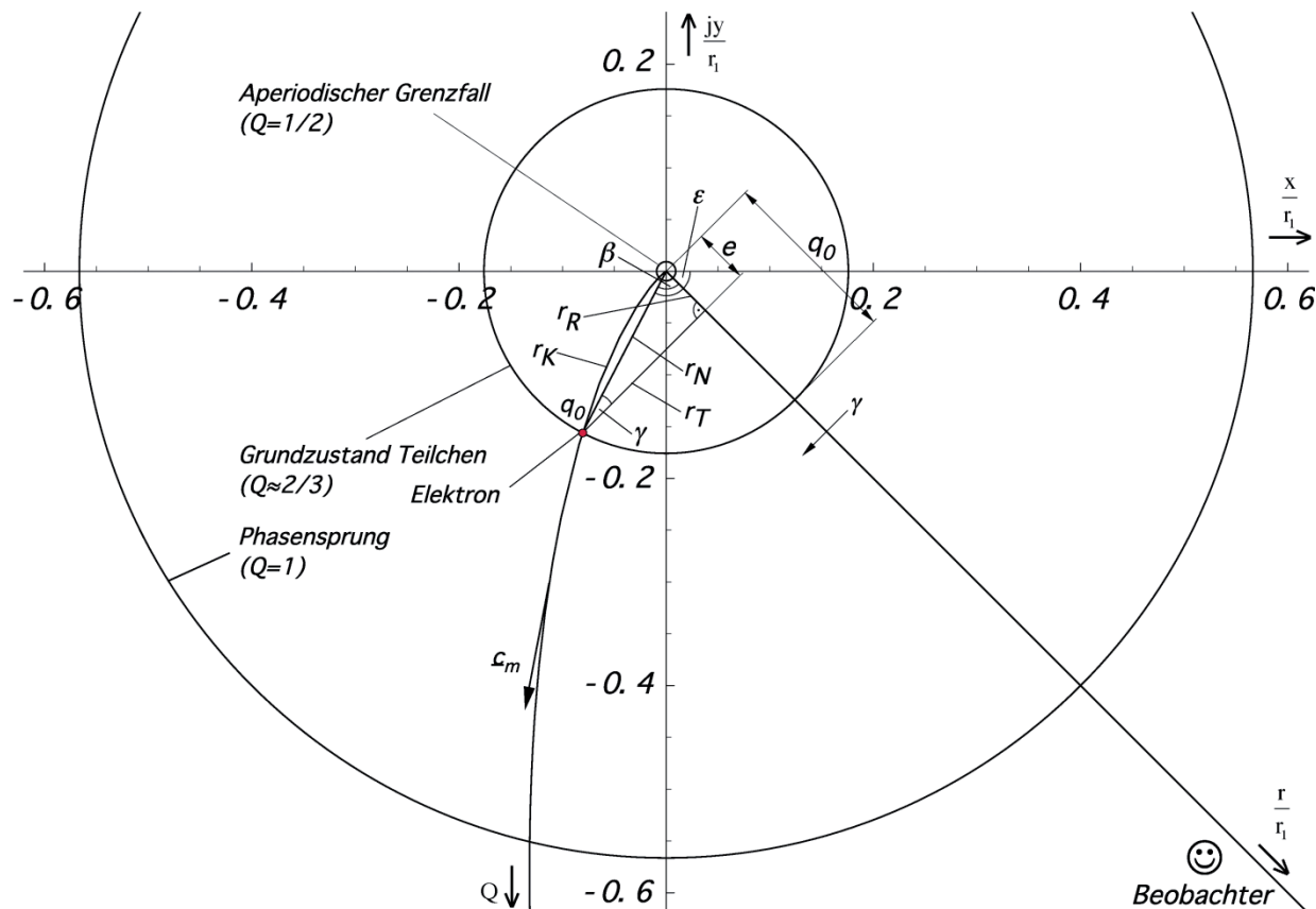
Bild 115 Verhältnis von Elektronenladung und Ladung des MLE im Phasenraum des Elektrons
