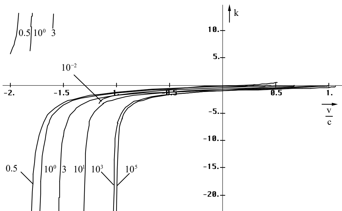
Bild 114 Relativistische Dopplerverschiebung (Wellenlänge) der Antineutrinos bei einer Güte von Q < 10^5
