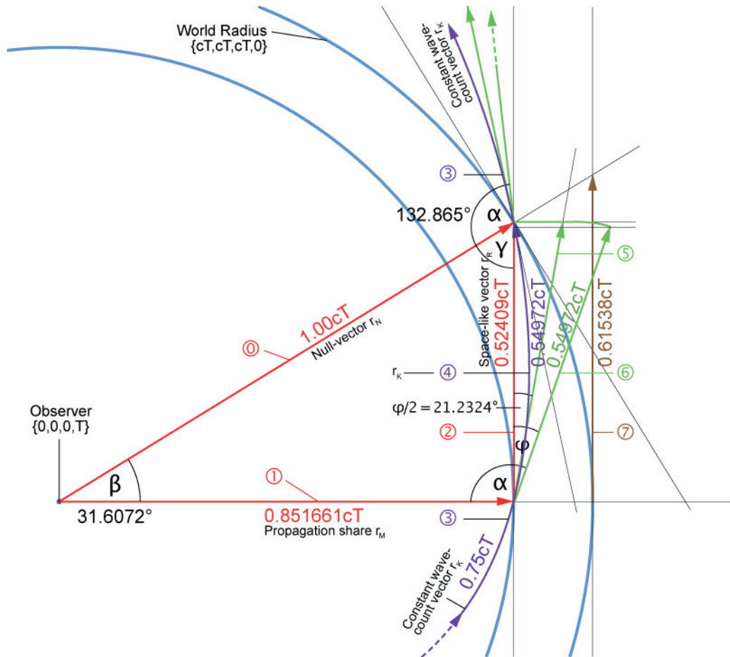
Bild 44 Expansionsgeschwindigkeit und Weltradius im Modell
