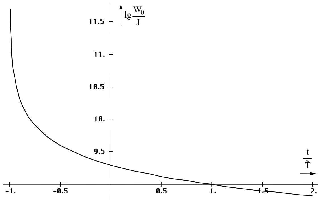
Bild 58 Energie des MINKOWSKISCHEN Linielements zeitliche Abhängigkeit
