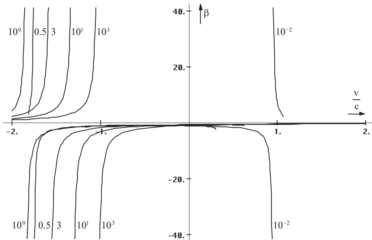
Bild 110 Relativistischer Dehnungsfaktor \beta_\alpha(v) für Antineutrinos
