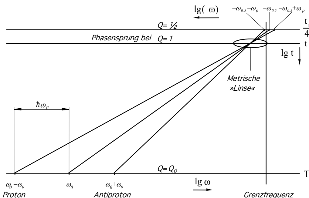
Bild 73 Masse-Rotverschiebung am Beispiel des Protons
