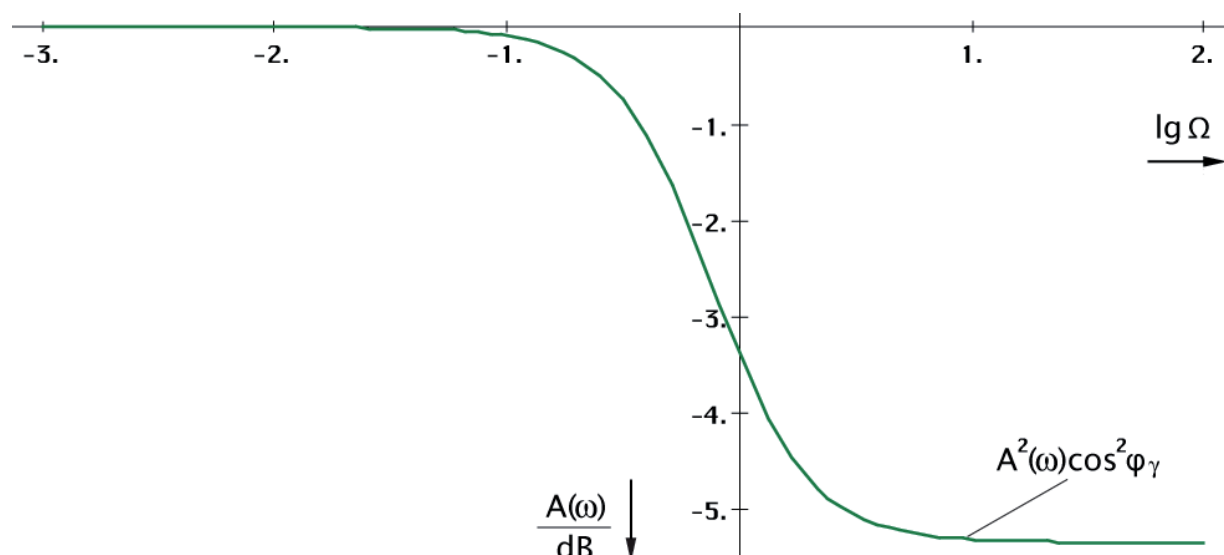
Bild 20 Frequenzgang für die Übertragung zum benachbarten MLE
