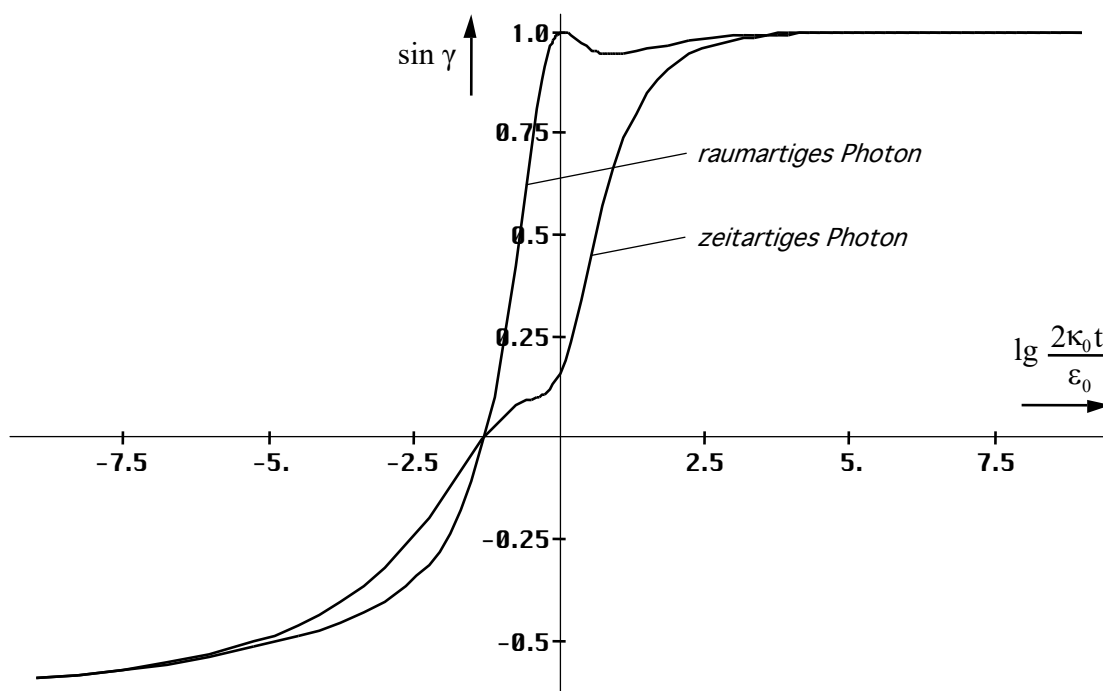
Bild 97 Verlauf der Funktion \sin \gamma des Schnittwinkels mit der Metrik für zeitartige (normale) und raumartige Photonen in der Nähe der Singularität
