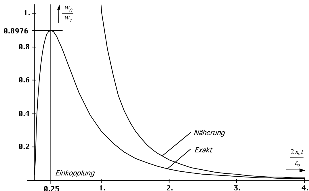
Bild 79 Zeitliche Abhängigkeit der Energiedichte des metrischen Wellenfeldes exakt und Näherung
