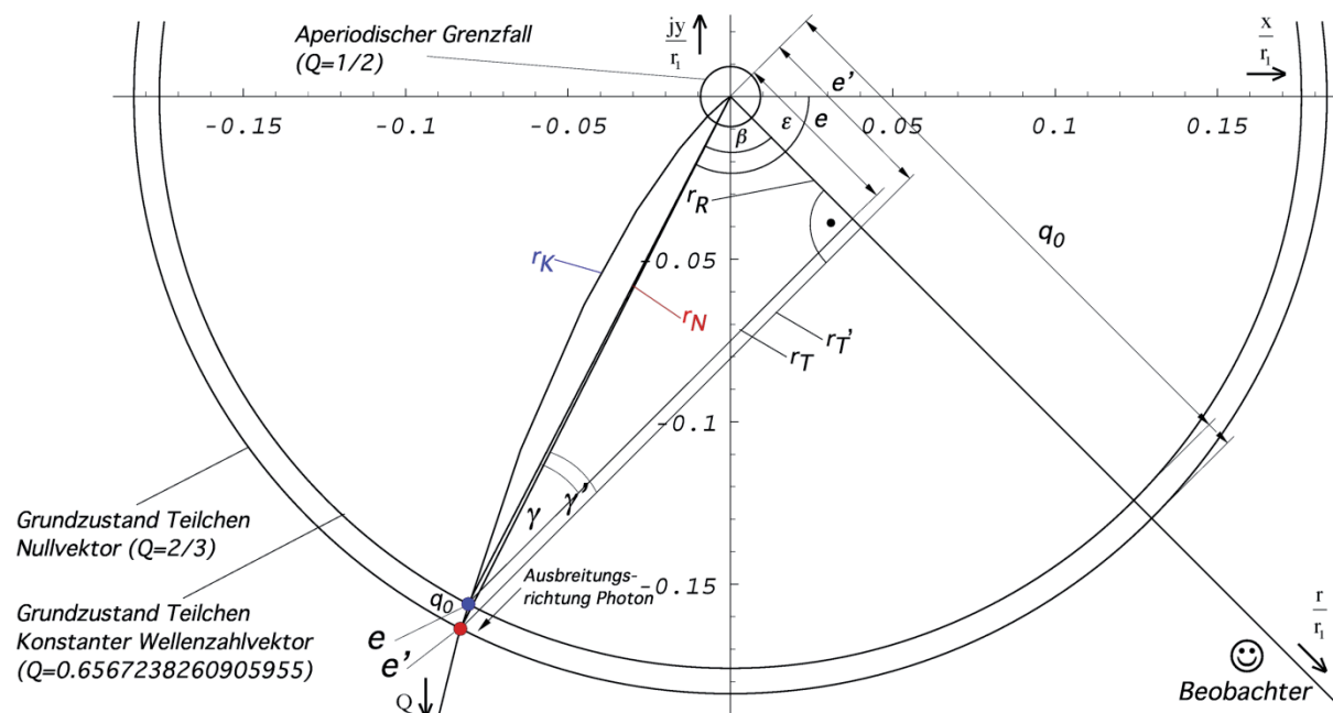
Bild 117 Verhältnis von Elektronenladung und Ladung des MLE im Phasenraum des Elektrons (größerer Maßstab)
