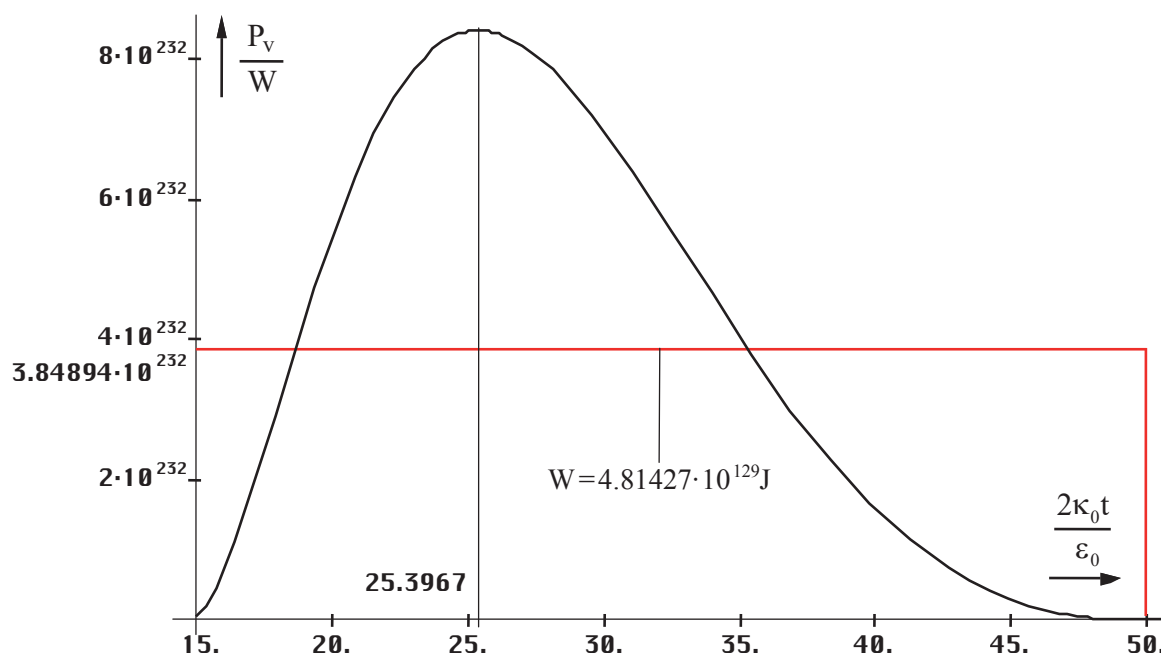
Bild 64 Verlustleistung des MINKOWSKISCHEN Linienelements während des zweiten Maximums
