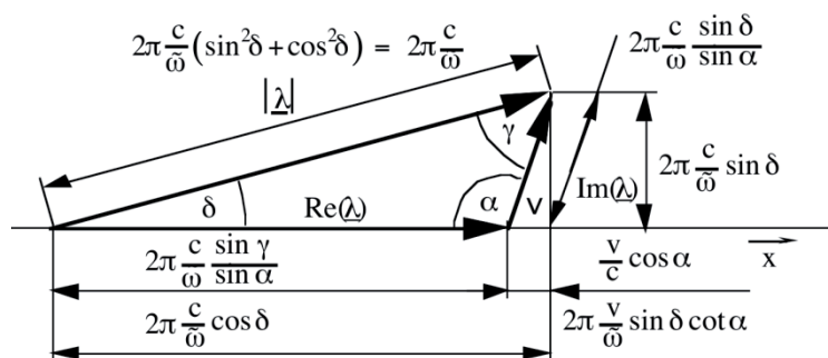
Bild 104 Wirkung des relativistischen Dehnungsfaktors \beta
