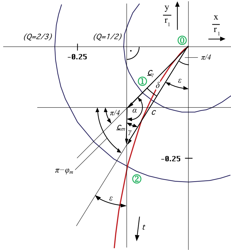
Bild 94 Vektorielle Geschwindigkeitsaddition bei Photonen in der Nähe der Singularität
