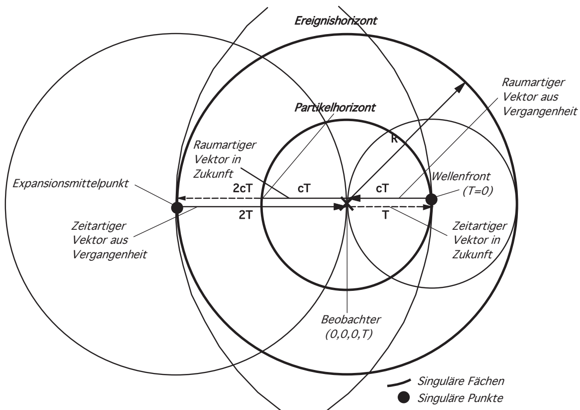
Bild 69 Weltmodell mit Verlauf raumartiger und zeitartiger Vektoren
