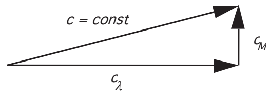
Bild 34 Ausbreitungsgeschwindigkeit der Metrik und einer überlagerten elektromagnetischen Welle
