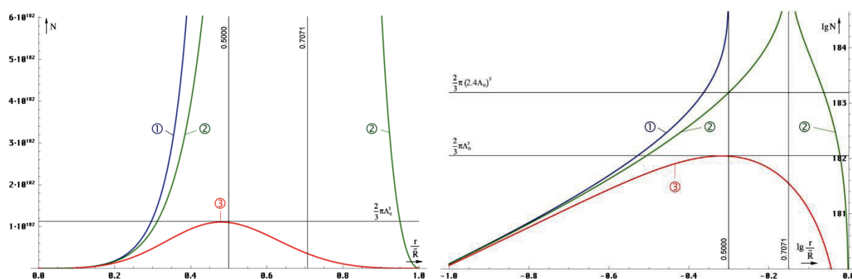
Bild 45 Anzahl Linienelemente in Abhängigkeit vom Radius linear und logarithmisch
