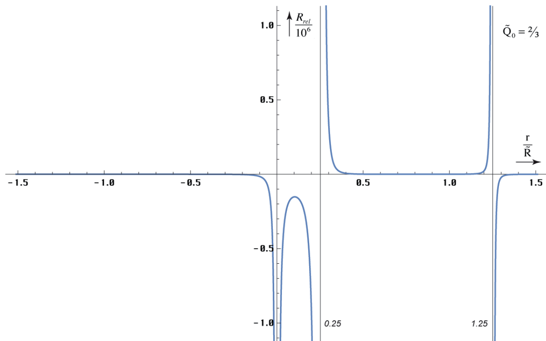
Bild 135 Relative skalare Krümmung für den Fall Q_0 = 2/3
