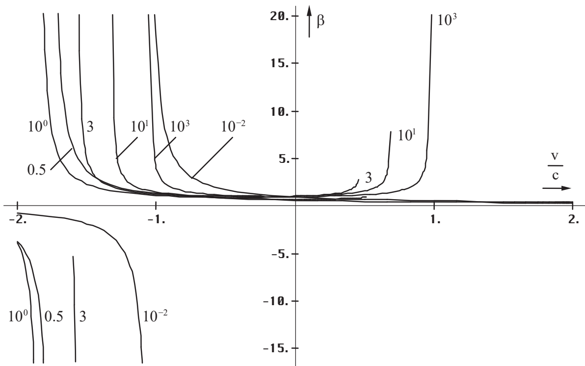
Bild 108 Relativistischer Dehnungsfaktor \beta_\alpha(v) für raumartige Photonen
