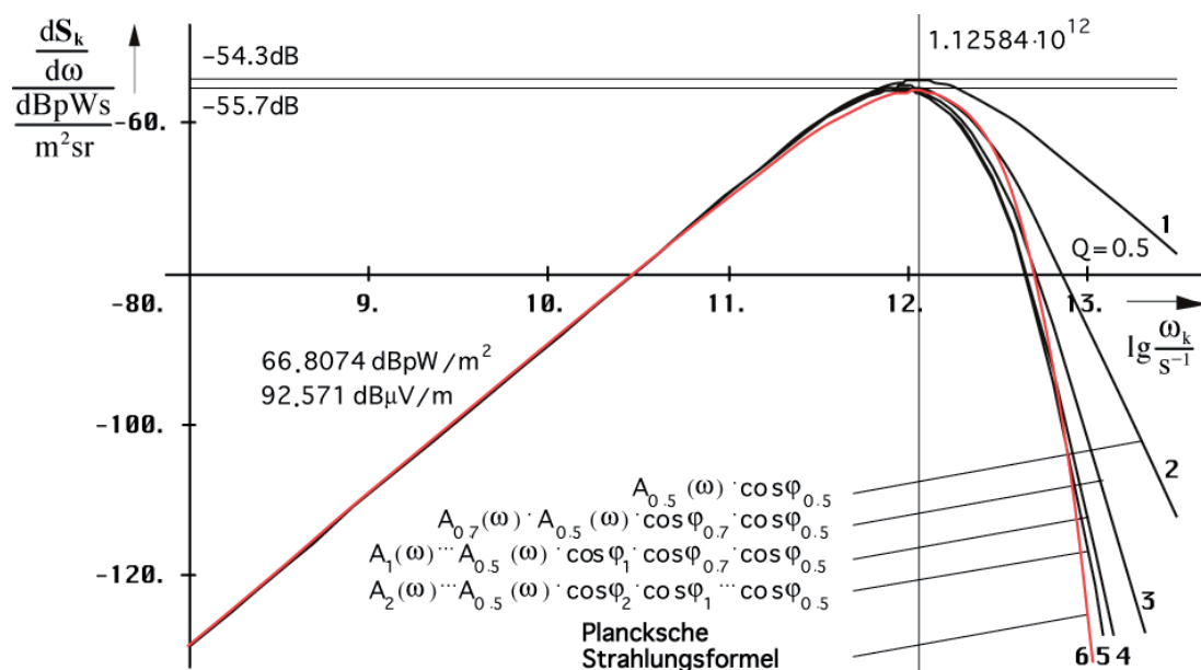
Bild 67 Intensität der kosmologischen Hintergrundstrahlung mit Approximation
