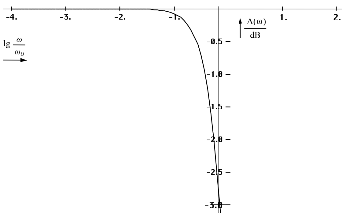
Bild 86 Normierte Spektralfunktion |X_n(j\omega)| der elektrischen bzw. magnetischen Feldstärke des Urimpulses (logarithmischer Maßstab)
