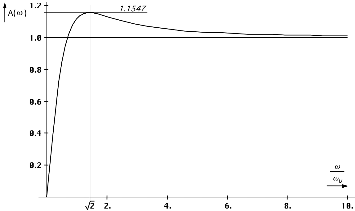
Bild 87 Energetisches Spektrum der elektrischen bzw. magnetischen Feldstärke des Urimpulses
