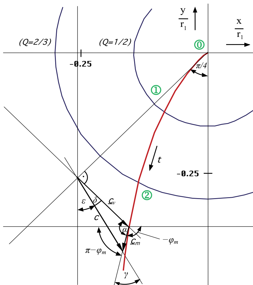
Bild 98 Vektorielle Geschwindigkeitsaddition bei Neutrinos in der Nähe der Singularität
