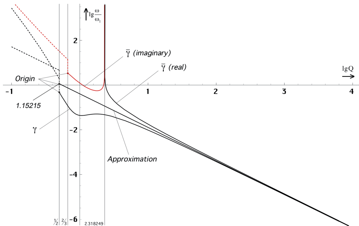
Bild 100 Rotverschiebung von Photonen exakt und Näherung
