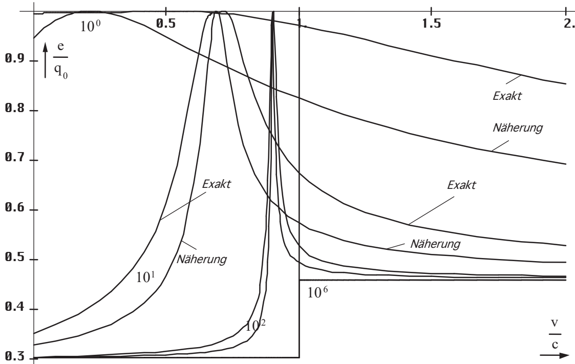
Bild 121 Verhältnis von Elektronenladung zur Ladung des MINKOWSKISCHEN Linielements als Funktion von Güte und Geschwindigkeit v=v_M + c_M
