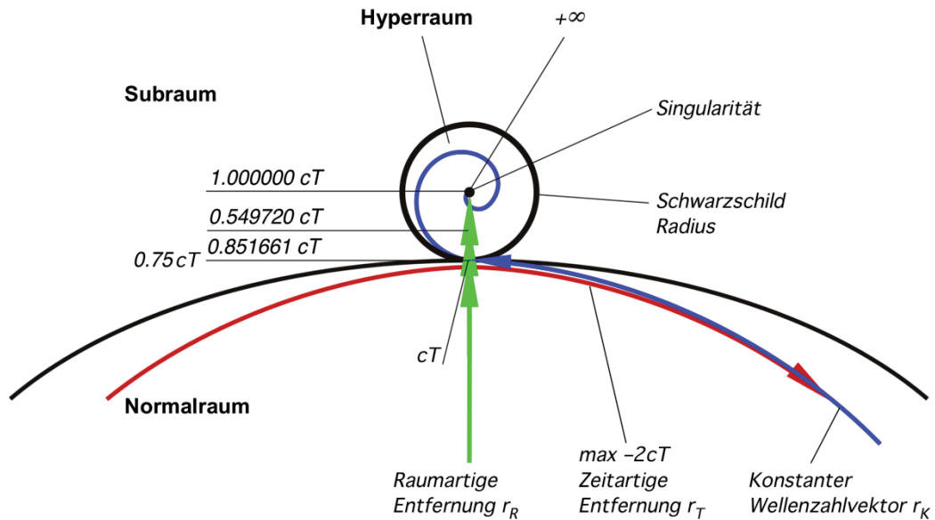
Bild 141 Verhältnisse am Rande des Universums
