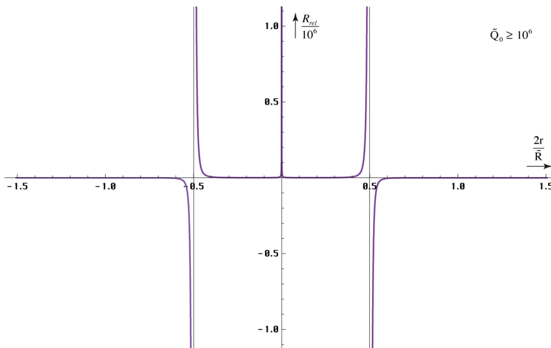
Bild 134 Relative skalare Krümmung für den Standardfall Q_0 > 10^6
