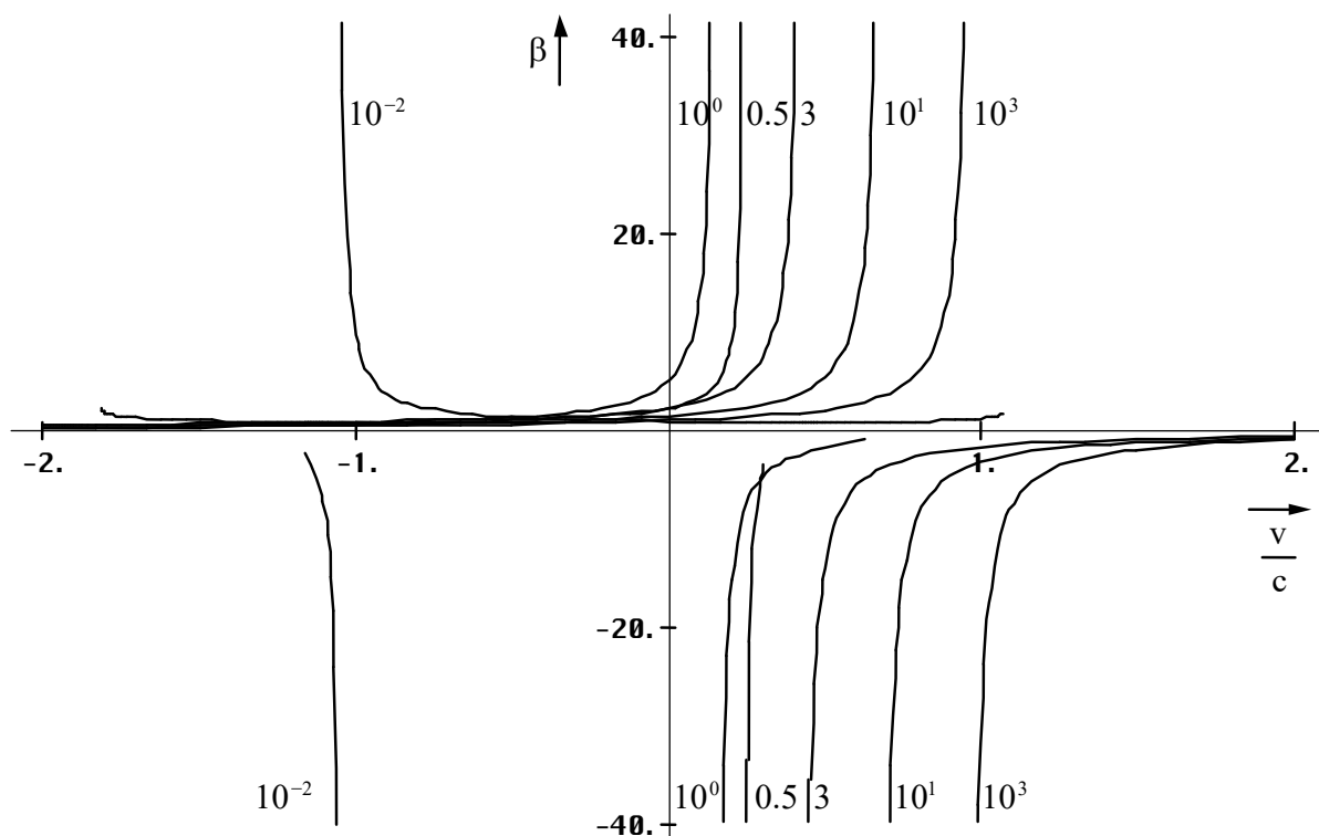
Bild 109 Relativistischer Dehnungsfaktor \beta_\alpha(v) für Neutrinos
