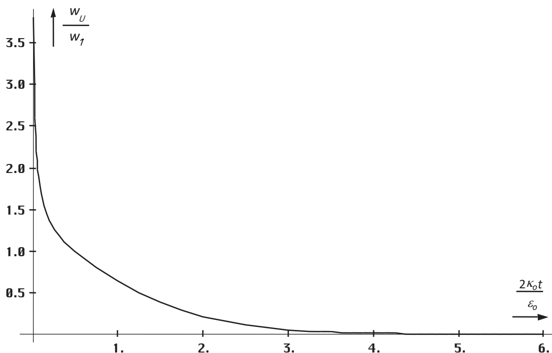
Bild 91 Mittlere Energiedichte des Uripulses
