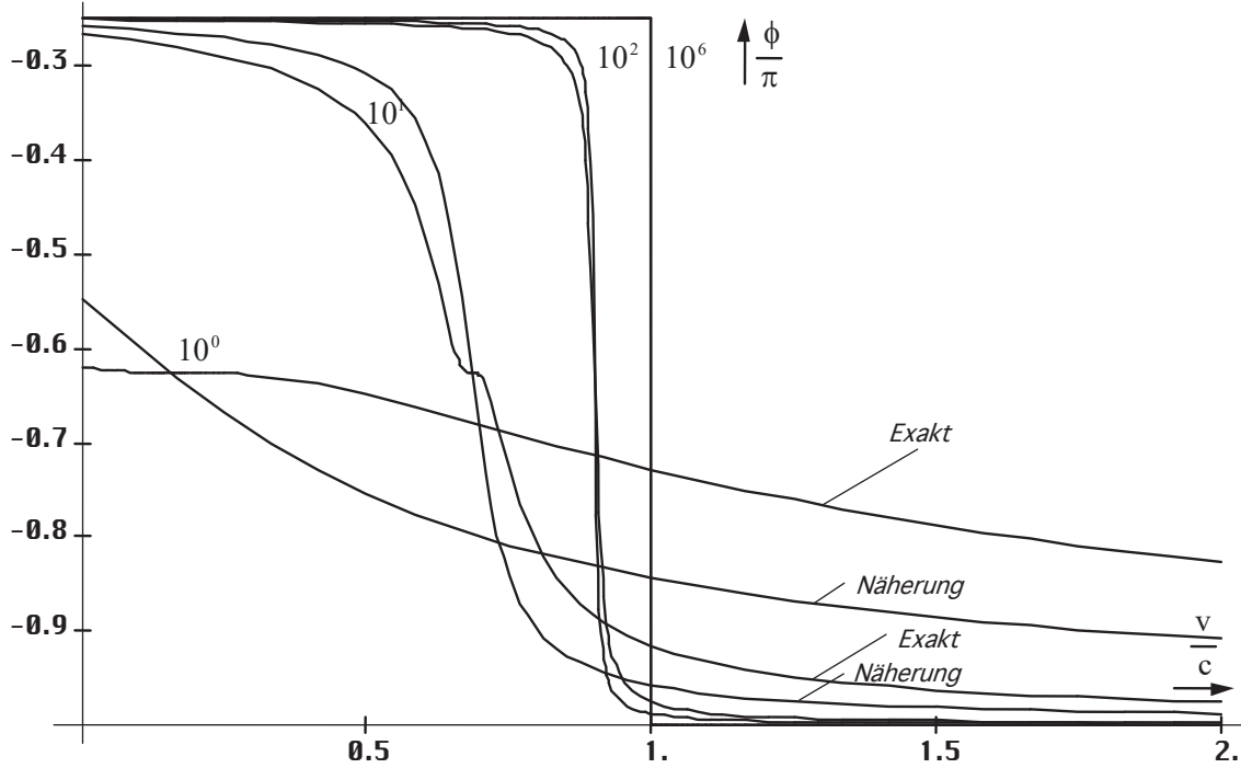
Bild 120 Phasenwinkel \phi des Beobachters als Funktion der Geschwindigkeit v=v_M + c_M
