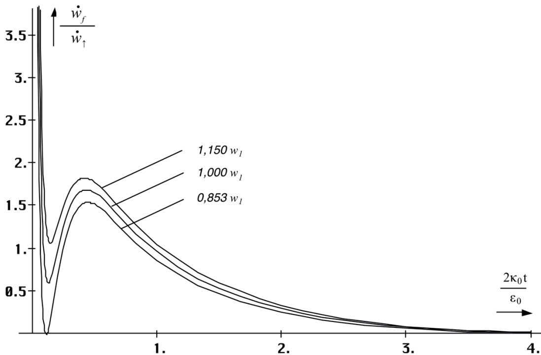
Bild 92 Leistungsdichte Fermionenerzeugung beim Urimpuls
