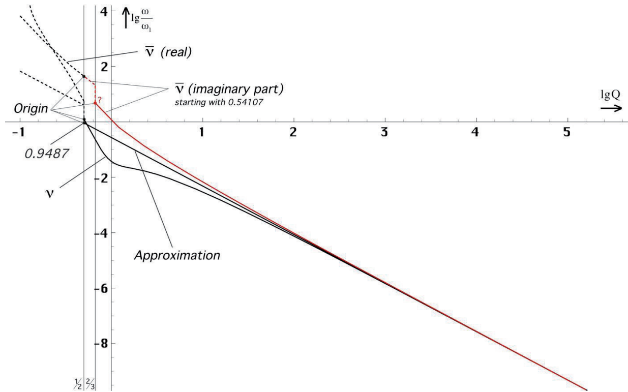
Bild 101 Rotverschiebung von Neutrinos exakt und Näherung
