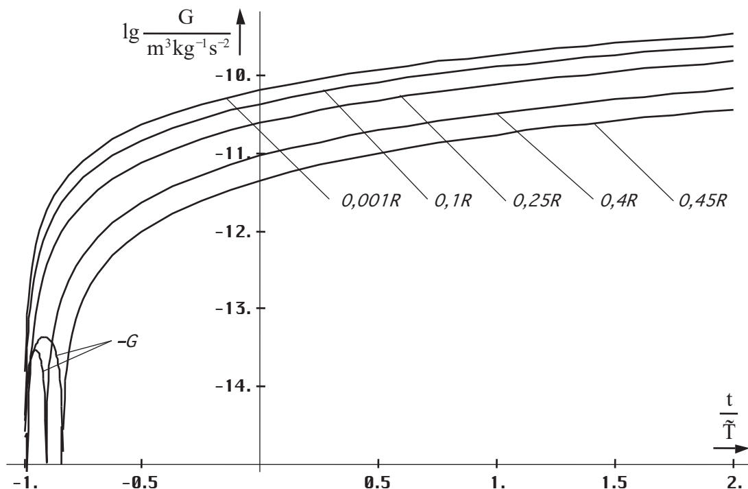
Bild 125 Zeitlicher Verlauf der lokalen Gravitationskonstante im Abstand r bei konstantem Wellenzahlvektor
