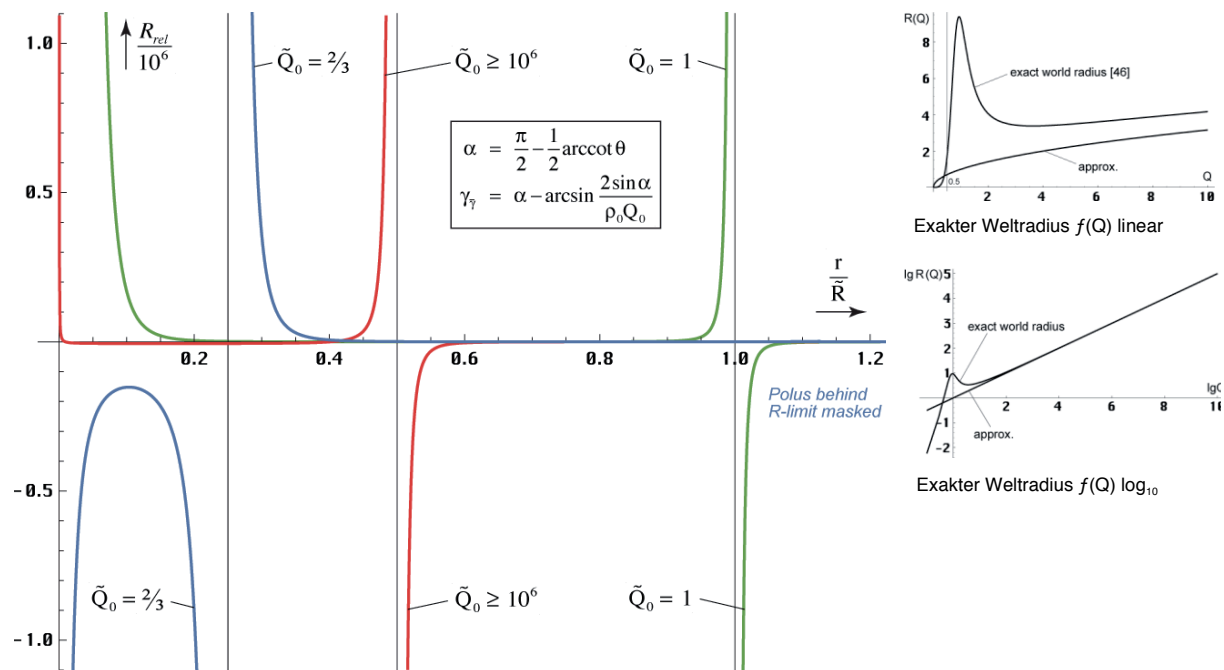
Bild 133 Relative skalare Krümmung für verschiedene Ausgangsgütewerte
