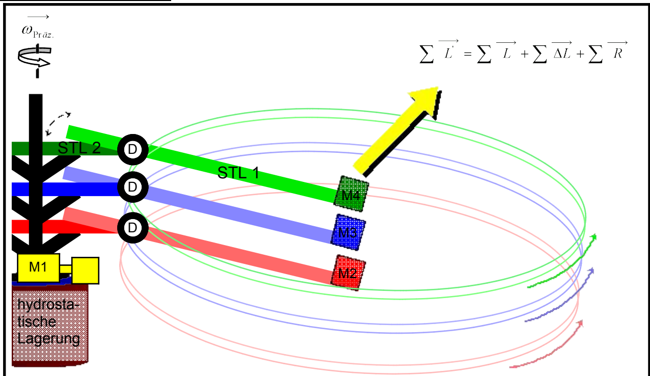
Abbildung 13 : RS1B2- Wandler
