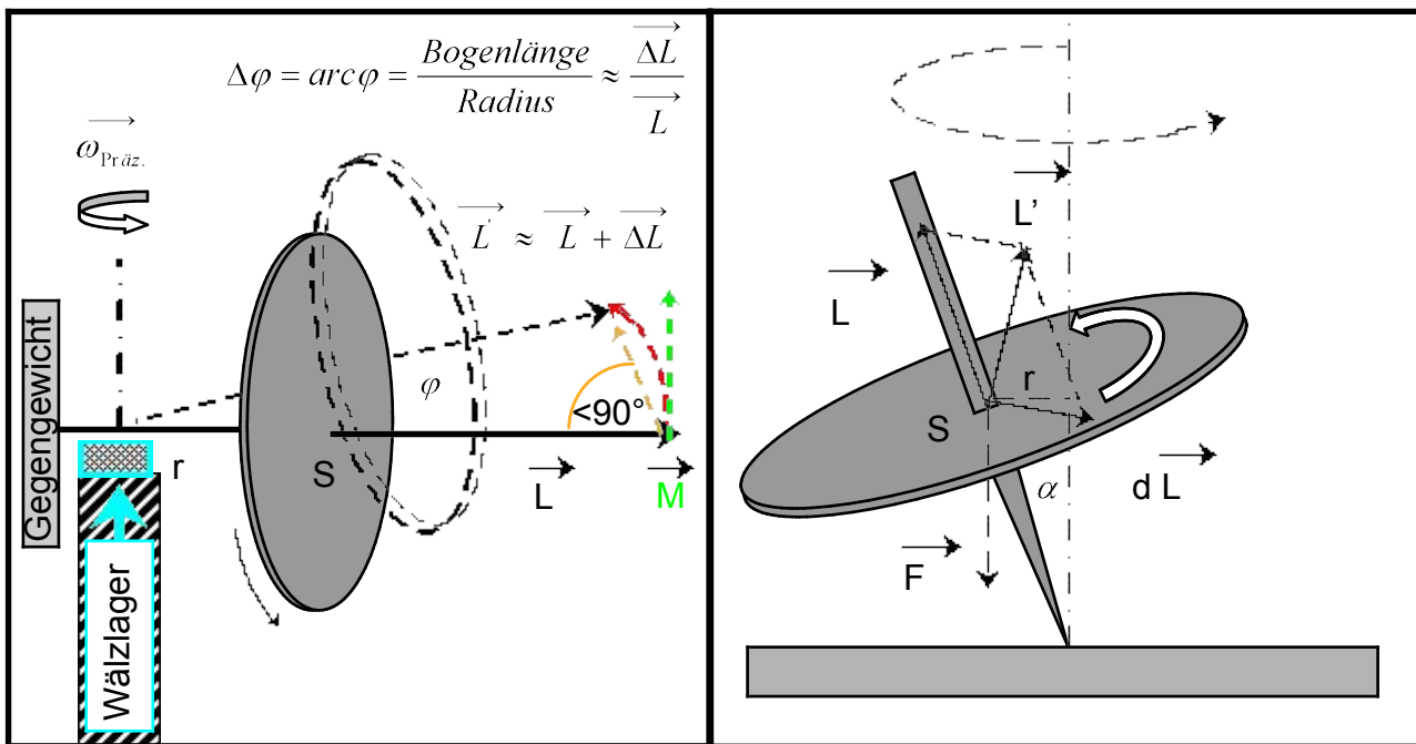
Abbildung 7: kippender Kreisel 1 Freiheitsgrad
