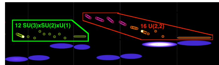
8 Fermion AntiParticles
