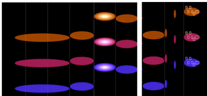
M4 M4 x CP2 Kaluza-Klein Quaternionic Spacetime
