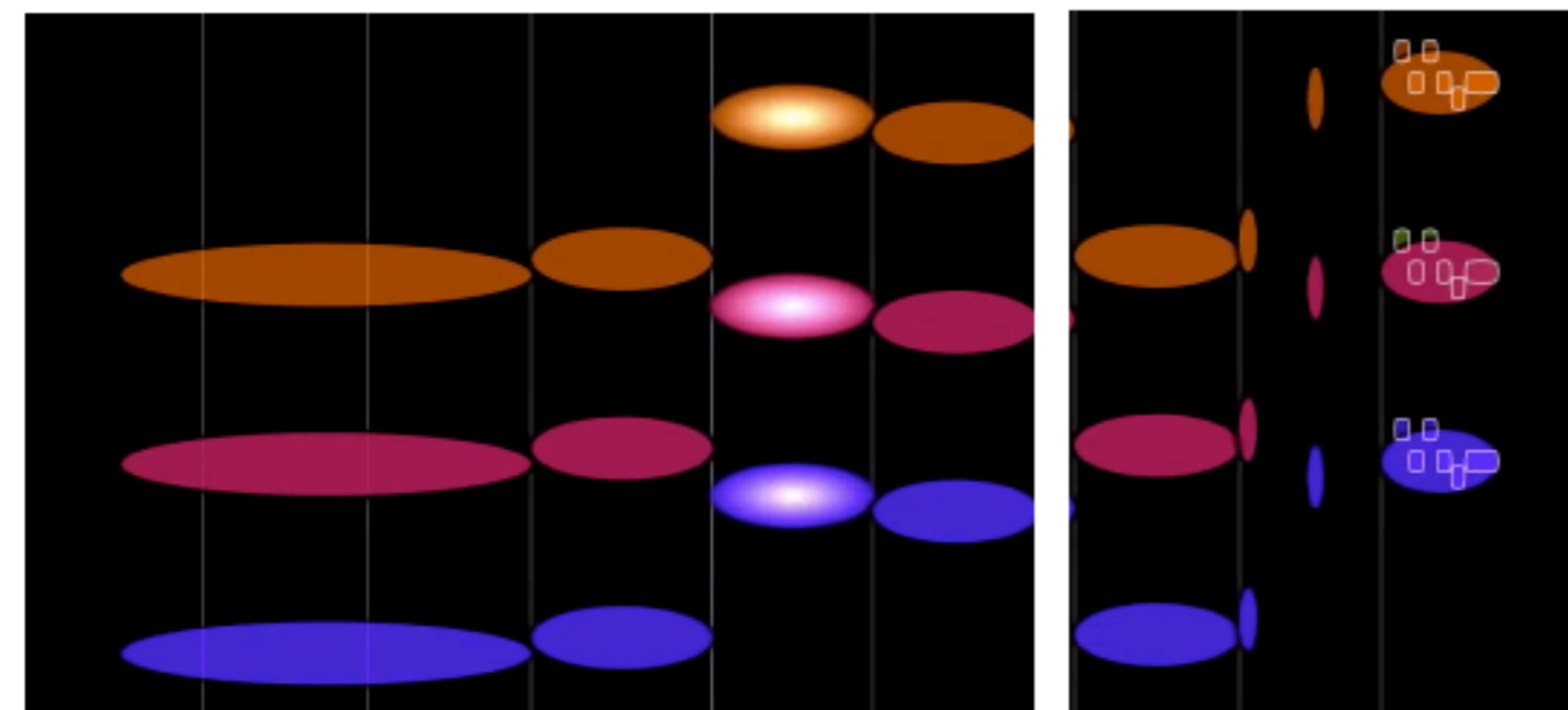
M4 M4 x CP2 Kaluza-Klein Quaternionic Spacetime
