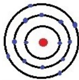
Bohr
