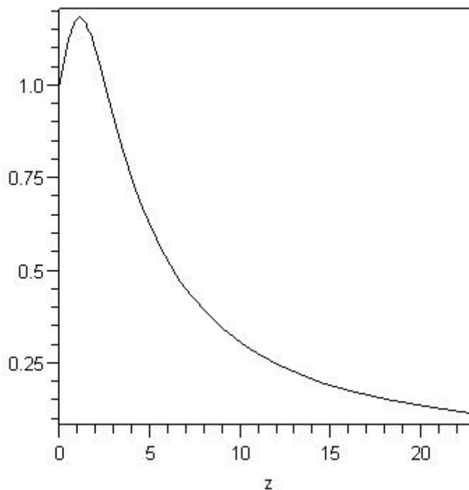
Рисунок 4. Зависимость отношения параметра Хаббла в \Lambda\text{CDM} -модели к его значению в данной теории.
