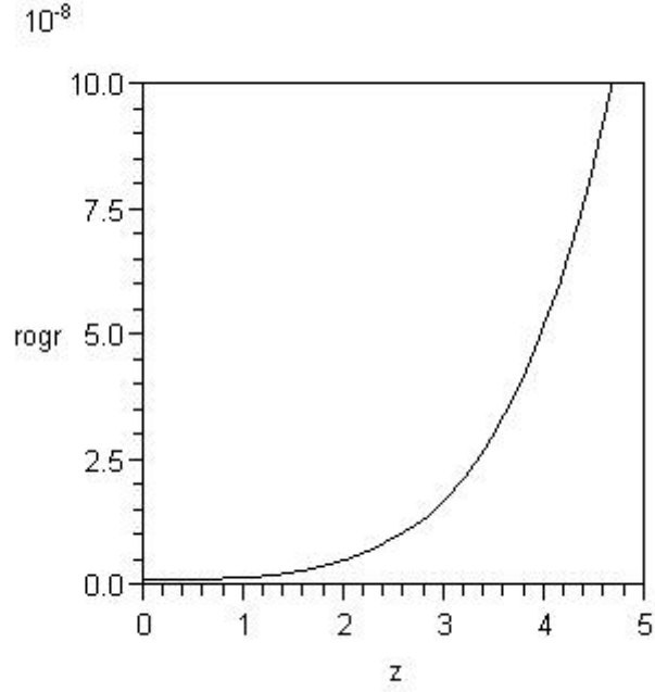
Рисунок 7. Зависимость плотности энергии гравитационного поля \rho_{gr} ( 10^{-8} Дж·м -3 ) от красного смещения в месте нахождения наблюдаемых гравитационно-связанных объектов, \rho_{gr\max} = 2 \cdot 10^{49} Дж·м -3 .
