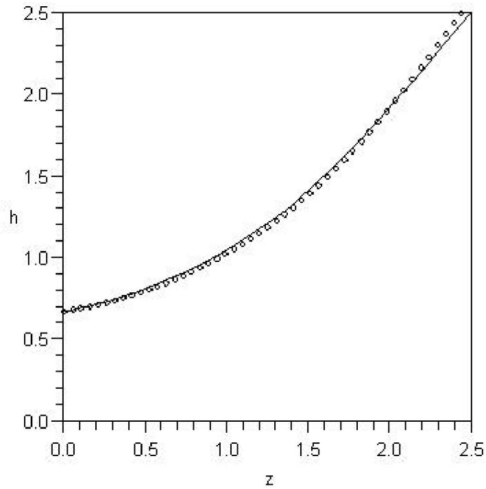
Рисунок 8. Результаты расчета зависимости параметра Хаббла ( H=100h \text{ км}\cdot\text{с}^{-1}\cdot\text{Мпс}^{-1} ) от красного смещения с учетом (сплошная линия) и без учета (точки) наличия материи.
