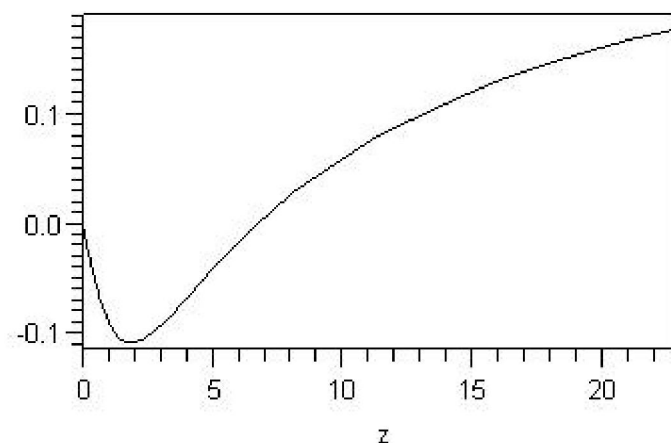
Рисунок 2. Отклонение от единицы отношения расстояний, вычисленных по OTO и данной теории, в зависимости от величины красного смещения.
