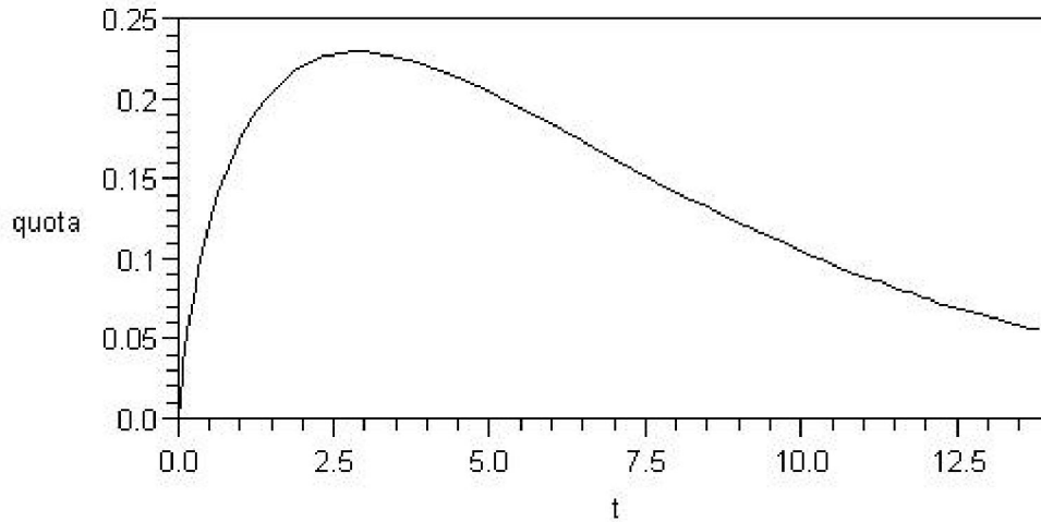
Рисунок 6. Зависимость отношения средней плотности энергии материи к плотности энергии во Вселенной в зависимости от времени (в миллиардах лет), \rho_{grmax} = 2 \cdot 10^{49} Дж·м -3 .
