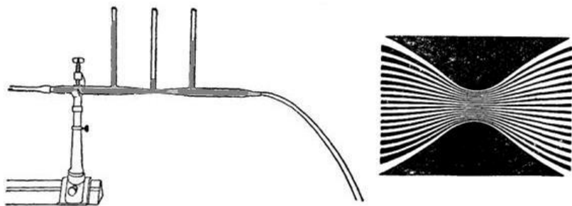
Распределение статического давления при течении через сужение. Три вертикальные стеклянные трубки служат водяными манометрами.
