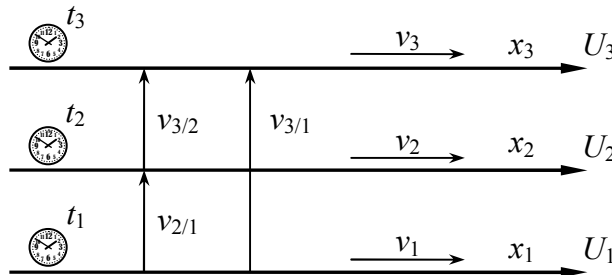
Rys. 5. Układy inercyjne U_1 , U_2 , U_3 poruszające się względem UFR z prędkościami v_1 , v_2 , v_3 .
