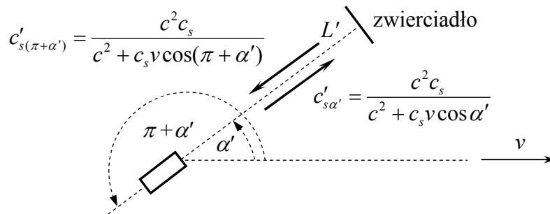
Fig. 4. Prędkości światła w eksperymentach Michelson'a-Morley'a.
