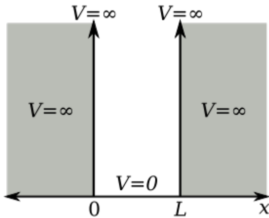
Figura 1. Esquema del pozo de potencial unidimensional.
