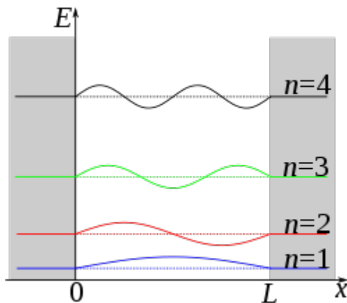
Figura 2. Representación de los primeros 4 niveles de energía posibles. Autor de la imagen: Papa November, bajo licencia CC BY-SA 3.0 .
