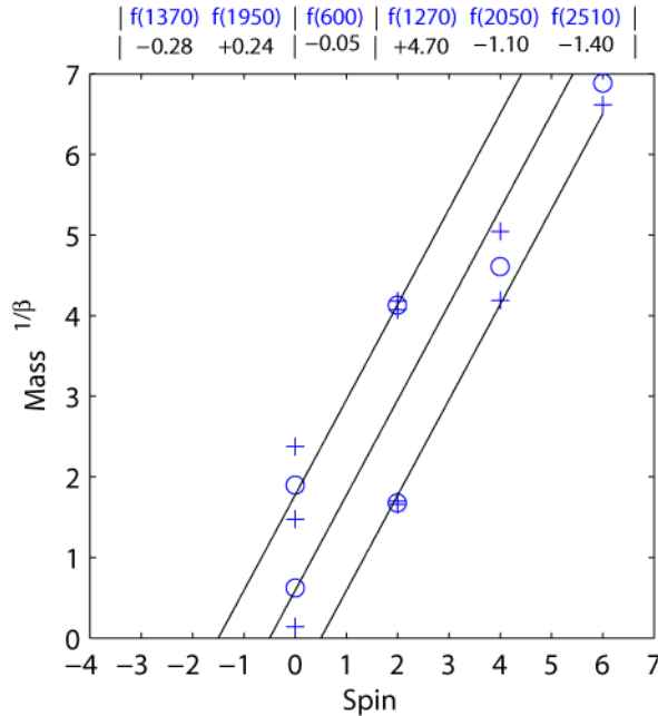
FIGURE 23. Positive parity f1
