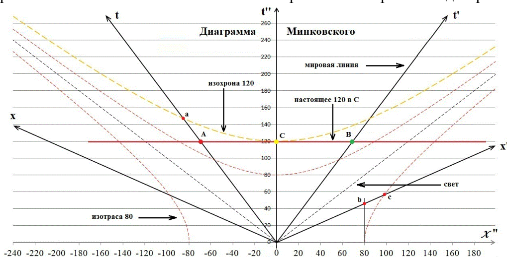
Рис.1 Диаграмма Минковского для двух движущихся систем отсчета А и В с точки зрения средней, неподвижной системы С в момент времени 120 секунд от начала движения.
