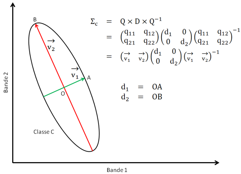
figure I.15 : Construction d'un ellipsoïde représentant une classe C suivant deux dimensions
