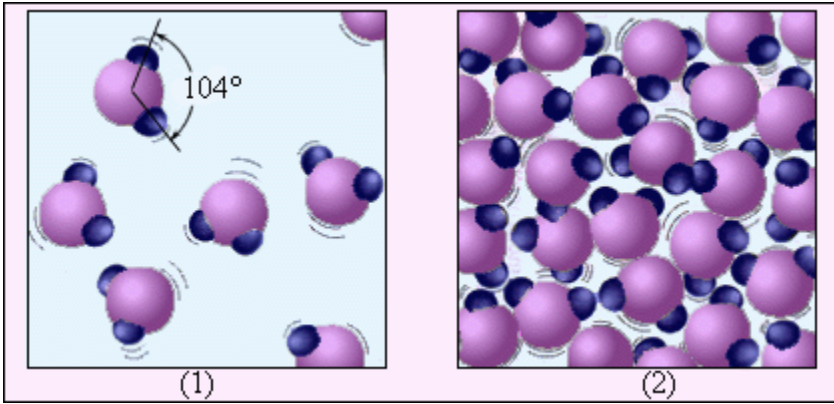
Рис. 2 (из Википедии). Водяной пар (1) и вода (2). Молекулы воды увеличены примерно в 5 \cdot 10^7 раз.
