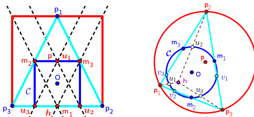
Figura 8: Demostración del Teorema 3.4
