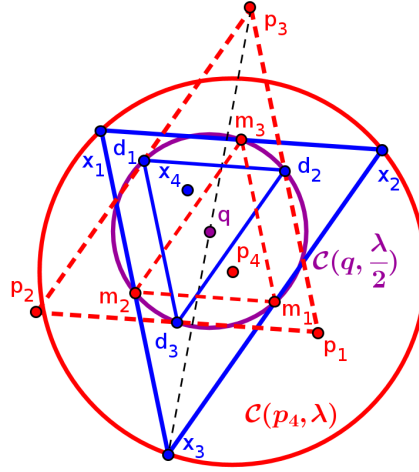
Figura 2: Demostración de los ítem 1 y 2, Lema 3.1
