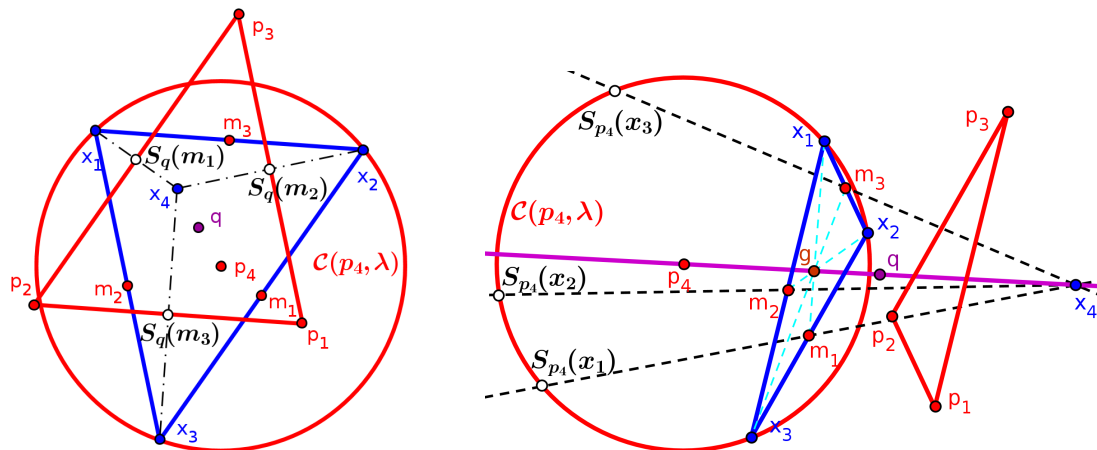
Figura 4: Demostración del Lema 3.2
