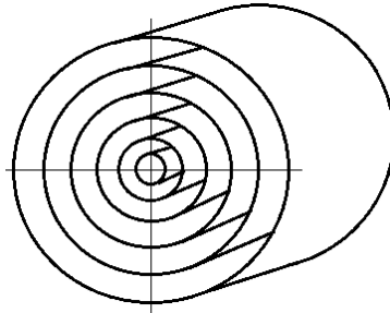
Рис.8. Поперечное сечение тора Архимеда может иметь вид концентрических кругов
