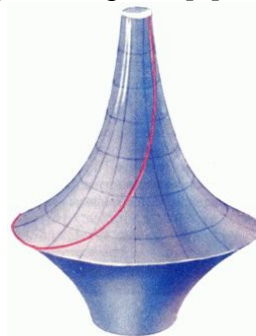
Рис.1. Псевдосфера Бельтрами (нижняя часть симметрична верхней)
