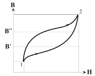
Рис.4. Цикл магнитного двигателя
