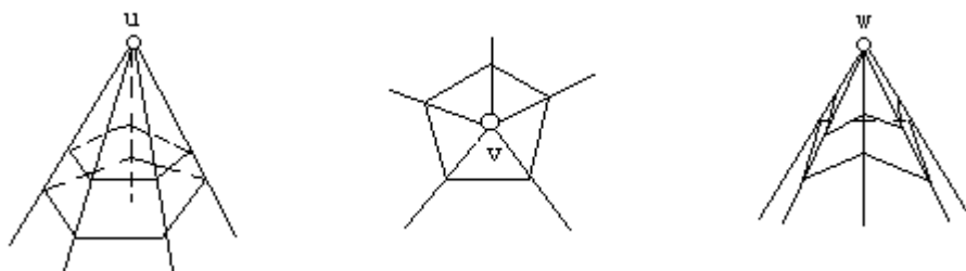
图 3.6. 椭圆点、欧氏点和双曲点在 3- 维空间的实现
